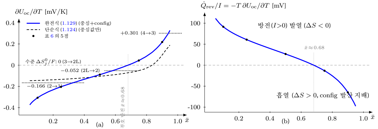
Figure 22: 완전식이 만드는 하프셀 엔트로피 계수와 가역 발열의 실제산 곡선 — 좌표는 식 그대로의 수치 평가다(4-전이 staging 입력: 표 3의 \Delta S_j^0 , w_j=RT/F ( n_j=1 ), 298.15 K; 각 \bar{x} 에서 전하 보존 음함수 (1.119)를 풀어 U_{oc} 를 얻은 뒤 평가). (a) \partial U_{oc}/\partial T(\bar{x}) — 파란 실선 = 완전식 (1.129)(중심 표준값+분포 config), 검은 파선 = 단순식 (1.124)(중심값만) 이고 둘의 차가 봉우리 내부 config 항이다(파생 B). 점선 수평선은 전이별 수준 \Delta S_j^0/F — 곡선이 전이 경계마다 계단 없이 인접 수준 사이를 연속으로 지난다(파생 A의 연속 블렌드). ●는 표 6의 다섯 점과 일치하며 \bar{x}=0.25 값이 계산 예제 (§1.18.2)의 -0.204 / 단순식 -0.134 mV/K 다. (b) 가역 발열 \dot{Q}_{rev}/I = -T\partial U_{oc}/\partial T (식 (1.128)) — \bar{x} \approx 0.68 에서 방전 발열이 흡열로 스스로 반전한다(임의 함수·외부 스위치 없이 분포만으로). 완전식 곡선은 폭의 열적 서식 w_j=n_jRT/F 를 전제하며, 실측 폭이 T -동결에 가까우면 단순식이 보수적 기준이다 (§1.15.4).
