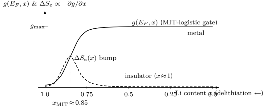
Figure 8: LCO 전자 엔트로피의 MIT-logistic 게이트(신규). 실선 = g(E_F, x) (식 (1.36)): x \approx 1 절연체에서 \approx 0 , 탈리튬화로 x_{MIT} \approx 0.85 부근에서 metal 의 g_{max} = 13 \text{ e/eV} 로 켜진다. 파선 = 탈리튬화 시 방출되는 부분물 전자 엔트로피 |\Delta S_e| = -\partial S_e / \partial x \propto -\partial g / \partial x > 0 (식 (1.34)·달헌식 (1.37); 삽입 기준 \Delta S_e = \partial S_e / \partial x < 0 의 절댓값으로, x_{MIT} 에서 \sigma(1 - \sigma) 가 최대): 천이 중심의 국소 봉우리다 — 작지만(O3 부분물 \approx 0.18 k_B/\text{atom} ) MIT 구간에만 켜지는 게이트라 config 단독으로 대체 불가. \Delta S_{e,j} \propto T 라 다른 항과 달리 전자 기여의 \partial U / \partial T 가 T 에 선형 (§1.6.2; U-이동은 \propto T^2 ). 흑연엔 이 봉우리가 없다( g(E_F) 변화 미미).
