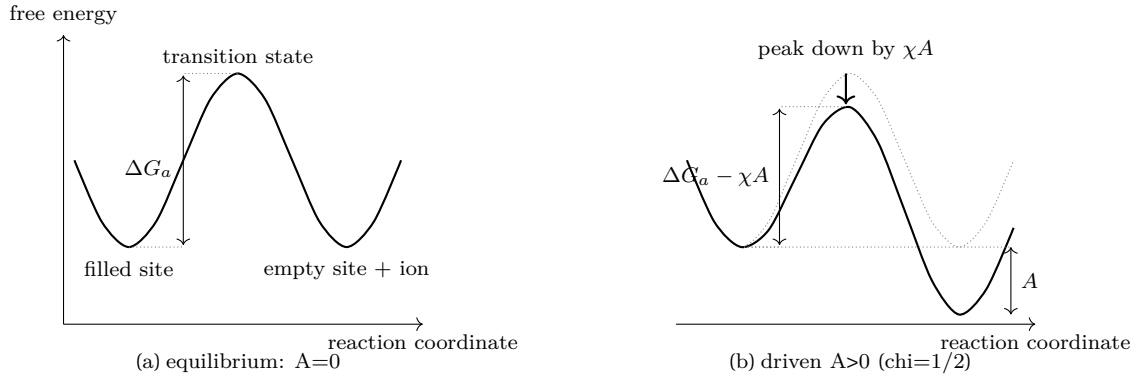
Figure 5: 활성화 장벽 그림 (신규). (a) 평형 — 두 골짜기 같은 높이, 속도는 Eyring 식. (b) 구동력 \mathcal{A}_j 가도착 골짜기를 내리면 정방향 장벽 \Delta G_a - \chi \mathcal{A} , 역방향 \Delta G_a + (1 - \chi) \mathcal{A} 로 비대칭 이동 (식 (1.26); 두 속도의 비가 식 (1.27) detailed balance). 점선은 (a). 온도는 분모 RT 로 진입. 이 그림이 식 (1.29) logistic 과 §1.8의 L_q 두 결과의 공통 출발점이다.
