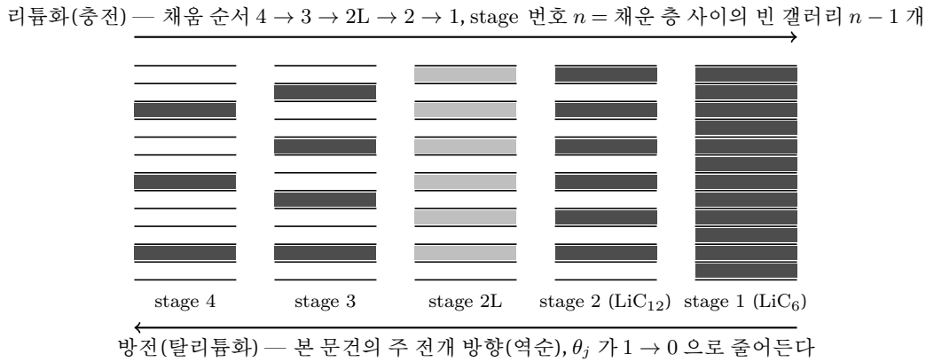
Figure 1: 흑연 staging의 갤러리 채움 도식. 수평선이 그려진 층, 음영 띠가 리튬이 든 층간 갤러리다. 채울수록 stage 번호가 줄어 stage 1(LiC 6 , 완전 채움)에 닿고, 각 stage 전이가 dQ/dV 에 peak 하나를 남긴다. stage 2L은 stage 2와 같은 주기이되 갤러리 안이 희박하고 면내 질서가 풀린(liquid-like) 단계라 열게 표시했다. 개념도이며 — 실제 채움은 갤러리 전체가 아니라 국소 도메인 단위로 진행되고 층의 굽힘을 동반한다(Daumas-Hérolld 그림, §1.3).
