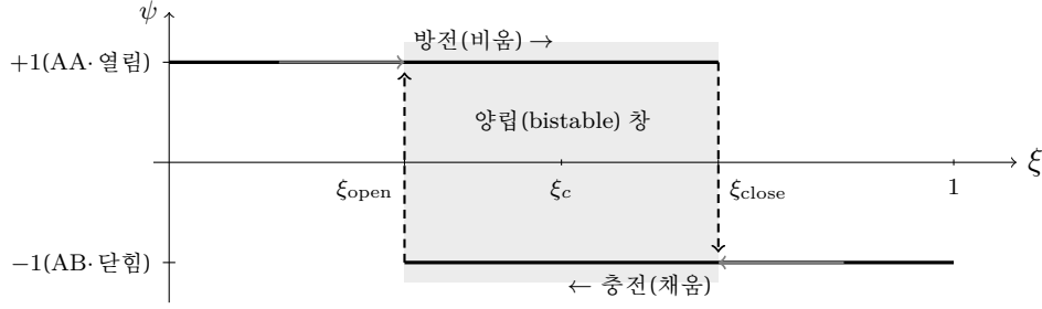
Figure 17: 적층 order parameter \psi 의 방향별 이력(식 (1.98)–(1.100); \xi_c = 0.5 , \Delta\xi_{\text{stack}} = 0.4 ). 충전 ( \xi 감소, 점유율 증가)은 닫힘 ( \psi = -1 )을 유지하다 \xi_{\text{open}} = 0.3 (점유율 70%)에서 열리고, 방전( \xi 증가)은 열림 ( \psi = +1 )을 \xi_{\text{close}} = 0.7 (점유율 30%)까지 버티다 닫는다(점선: 점화 점프; 가지는 \psi = \pm 1 로 이상화 — spinodal 부근 곡률은 생략). 두 임계 조성의 분리가 방향 비대칭이며, 음영의 bistable 창이 그 폭이다. B_j \rightarrow 0 에서 창이 닫혀 §1.13 의 대칭 그림으로 회수된다.
