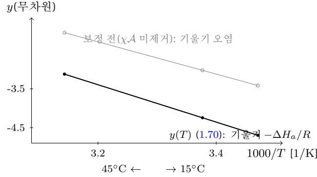
Figure 9: Arrhenius 회귀 (1.71) ( \Delta H_a = 40 kJ/mol, 절편 12, 세 온도 15/23/45°C). 검정: 보정된 y(T) (1.70) — 1/T 선형, 기울기 -\Delta H_a/R . 회색: 구동항 \chi A_j/RT 미제거 — offset 이 온도마다 달라 기울기 오염. S4 가 \chi 를 먼저 닫는 이유 (§1.15).
