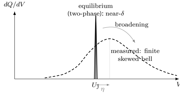
Figure 9: 두-상 전이의 평형 델타 vs 실측 중(신규). 솔리드 스파이크 = 두-상 전이의 평형 단일 입자 응답(이상적으로 무한히 좁은 선, near- \delta , 위치 = 평형 U_j ). 파선 = 실측 유한 폭의 치우친 종 — apparent- U_j = U_j + \eta 로 이동하고( \eta = 과전압), 유한율속 비대칭 꼬리 (§1.8.2(i)·입자 크기 분산(ii), 모델 L_V ·현상학적 w_j )가 한쪽 꼬리를 늘이며, 내재 RT/F 폭(iii)이 바닥을 깎다. 분포하는 것은 평형 U_j 가 아니라 \eta 이고, 그 폭은 현상학적 피팅 폭 w_j 와 동역학 길이 L_V 로 흡수된다 — 단상(고용체) 전이는 평형이 이미 종이라 이 그림이 필요 없다 (§1.8.1).
