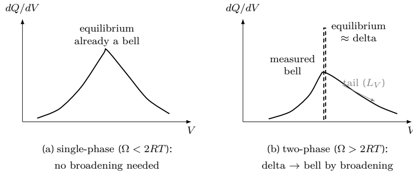
Figure 9: 평형 델타 vs 실측 종 (신규, broadening). (a) solid-solution 단상 전이( \Omega < 2RT )는 평형 등온선이 이미 폭 \sim n_j RT/F 의 종이라 broadening 이 불요하다 (§1.8.1). (b) 두-상 plateau 전이( \Omega > 2RT )는 평형 단일 입자가 델타(파선)에 가까운데, 실측 dQ/dV (실선)는 유한 폭의 넓어진 종이다 — 유한 율속 비대칭 꼬리(모델의 L_V , 식 (1.51))가 치우침을, 내재 RT/F 가 floor 를 만든다 (§1.8.2). 좁힘이 아니라 넓힘이며, 이 폭이 §1.5.1의 현상학적 자유 피팅 폭 w_j 다. 관측 중심은 \text{apparent-}U = U_j + \eta 이고 분포하는 것은 \eta (평형 U_j 아님).
