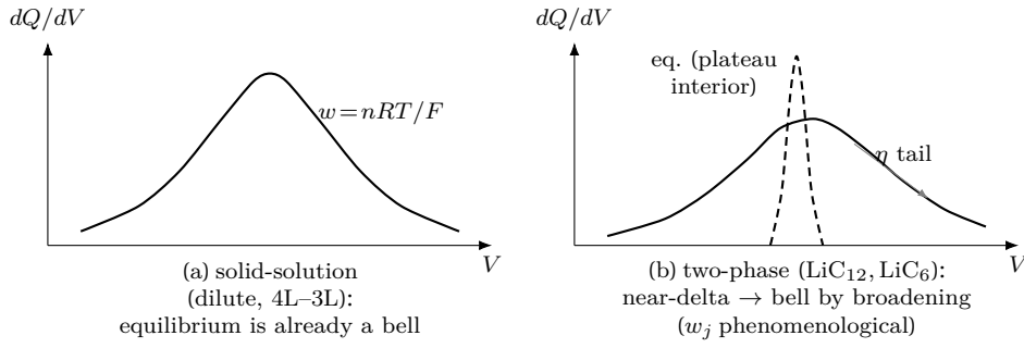
Figure 9: 평형 모양과 broadening(신규). (a) 연속 고용체 전이 — 평형 단일 입자 dQ/dV 가 이미 폭 n_j RT/F 의 중(식 (1.38)), broadening 불요. (b) 2상 전이 — 평형은 plateau 내부에서 거의 날카로운 선(파선, 단 양끝 단상 꼬리 탓에 폭이 정확히 0 은 아님)이나, 실측은 전류가 켜는 유한율속 비대칭 꼬리( \eta , §1.9 의 L_V , |I| \rightarrow 0 소멸)와 전류 무관한 가장자리 내재 폭( \sim RT/F )이 펼친 치우친 중(실선)이다. 후자의 폭 w_j 는 평형 예측이 아니라 broadening 이 정하는 현상학적 자유 피팅 폭이며, 이 중에서 평형 U_j ·반경 분포를 역산하지 않는다(§1.7.2(c)).
