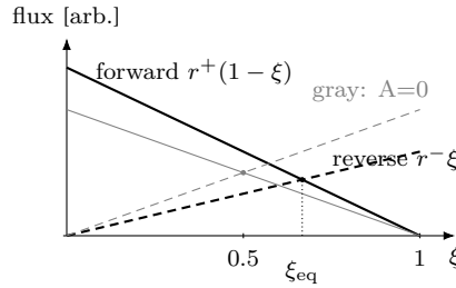
Figure 6: 정지점 유도 (신규). 정방향 플럭스 r^+(1 - \xi) (감소 직선)와 역방향 r^-\xi (증가 직선)의 교점이 정지점 \xi_{eq} (식 (1.27)). \mathcal{A} > 0 ( r^+ = 2r^- , 검정)이면 \xi_{eq} = 2/3 , \mathcal{A} = 0 (회색)이면 \frac{1}{2} — detailed balance (식 (1.26))가 평형을 정한다.
