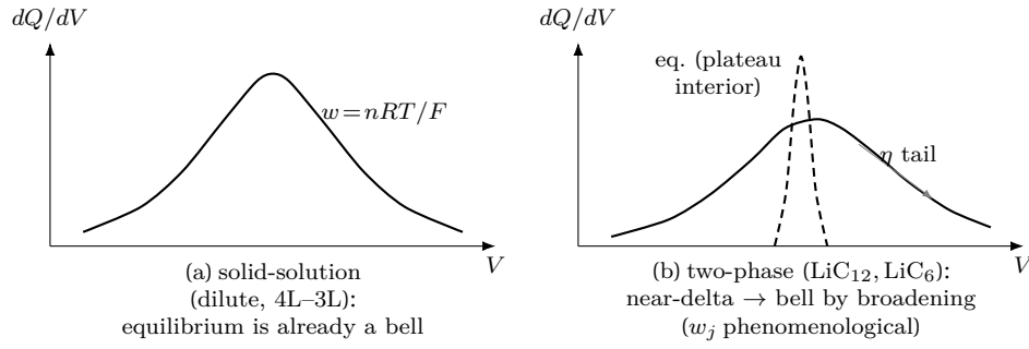
Figure 9: 평형 모양과 broadening(신규). (a) 연속 고용체 전이 — 평형 단일 입자 dQ/dV 가 이미 폭 n_j RT/F 의 종(식 (1.38)), broadening 불요. (b) 2상 전이 — 평형은 plateau 내부에서 거의 날카로운 선(파선, 단 양끝 단상 꼬리 탓에 폭이 정확히 0 은 아님)이나, 실측은 세 출처가 펼친 치우친 종(실선)이다: ① 전류가 켜는 유한율속 비대칭 꼬리( \eta , §1.9 의 L_V , |I| \rightarrow 0 소멸), ② 전류 무관한 가장자리 내재 폭( \sim RT/F ), ③ 입자 양상불의 전이 전위 분포 \rho(U_j) 를 forward 평균한 집합 통계역학 (식 (1.39); 비-크기 구조 무질서). 그 폭 w_j 는 평형 예측이 아니라 이 broadening 이 정하는 현상학적 자유 피팅 폭이며, 이 중에서 \rho(U_j) 를 역산하거나 입자 사이즈(반경)로 해석하지 않는다 (§1.7.2(c)).
