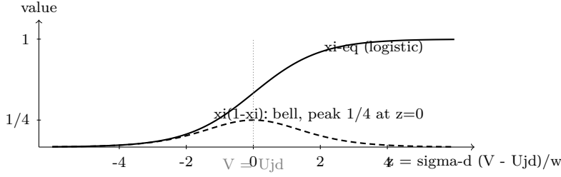
Figure 3: 평형 점유 logistic(실선, 식 (1.15))과 그 미분 종 \xi(1 - \xi) (파선, 식 (1.16); 신규 작성). 종은 중심 V = U_j^d(z = 0) 에서 최대 \frac{1}{4} , 폭 척도 w . 평형 peak(식 (1.18))은 이 종에 Q_j/w 를 곱한 것이므로 높이가 Q_j/(4w) ·면적 Q_j . \sigma_d 은 z 안에서 진행축만 거울로 바꾸고 종 자체(따라서 peak 부호)는 방향 불변이다.
