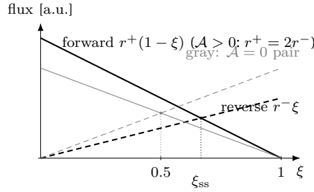
Figure 5: 정지점 (1.28): 정방향 r^+(1-\xi) (감소 직선)과 역방향 r^-\xi (증가 직선)의 교점(신규). A > 0 ( r^+ = 2r^- , 검정)이면 \xi_{ss} = 2/3 , A = 0 (회색)이면 \frac{1}{2} — 이 교점이 식 (1.29) logistic 으로 닫힌다.
