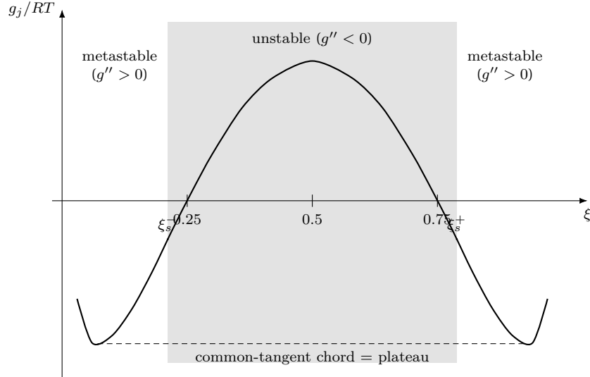
Figure 3: 자유에너지 (1.12) ( \Omega_j = 3RT ; 띠 경계는 spinodal (1.14) 실제산값, 신규 그림). 가운데 언덕은 g'' < 0 라 미소 요동에 즉시 무너지는 불안정 영역이고 그 경계 두 변곡점이 spinodal \xi_s^\pm , 옆은 양쪽 띠는 핵생성 장벽을 넘어야 하는 준안정(히스테리시스 무대)이다. 가장 낮은 현(공통 접선)이 평탄 전위 plateau — 좁은 dV 에 큰 dQ 가 몰리는 ICA peak 의 정체. 본 절은 두 spinodal 끝점의 전위 차로 분기 gap 을 닫는다.
