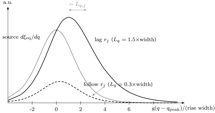
Figure 7: 일반해 (1.34) 의 기억 거동(신규). 점선 = 원천 d\xi_{eq}/dq . 파선( L_q = 0.3 \times 폭) = 축소 추종 (정점 \approx L_q \times 원천, 빠른 동역학 극한 L_q \rightarrow 0 에서 평형 추종 복귀). 실선( L_q = 1.5 \times 폭) = 기억이 상승부를 덮어 정점이 낮고 높으며 원천 포화 후 길이 L_q 로 지수 감쇠 — 상승부(추종)·꼬리(지수 기억)가 한 해의 두 얼굴. L_q 가 작으면 다음 절이 평형 종으로 환원되는 까닭이 이 그림이다.
