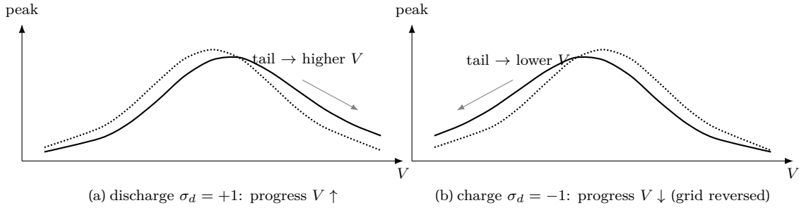
Figure 9: 인과 꼬리의 방향(v7-11 유래). 점선 = 평형 종 ( \xi_{eq}(1 - \xi_{eq})/w , 방향 불변). 실선 = peak_shape with tail. (a) 방전은 진행이 V \uparrow 라 꼬리가 높은 V 쪽으로 늘어진다(격자 그대로). (b) 충전은 진행이 V \downarrow 라 격자를 뒤집어 필터( \xi[:: -1] \cdots [:: -1] )해 꼬리가 낮은 V 쪽으로 — 방전의 거울. 두 경우 모두 peak 는 양수.
