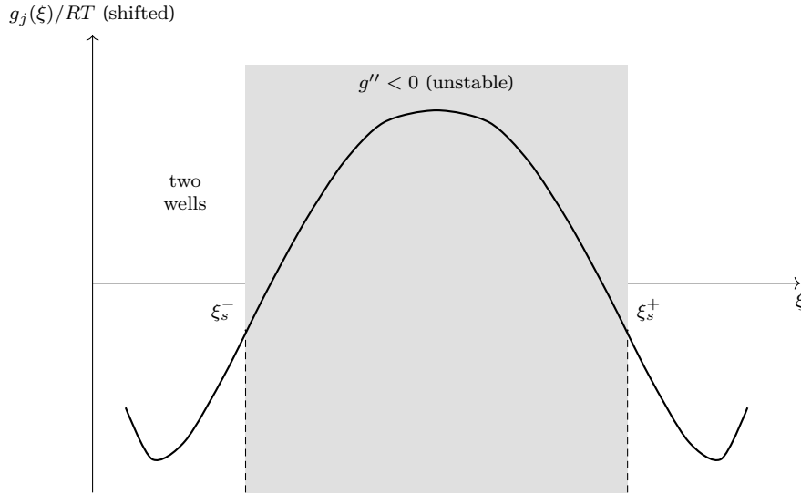
Figure 3: 격자기체 자유에너지 g_j(\xi) (식 (1.13), \Omega_j = 3RT ; 신규 그림). \Omega > 2RT 면 가운데가 언덕이 되어 양쪽에 골짜기 둘 — 음영 때 ( g'' < 0 , 식 (1.14))가 변곡점 \xi_s^\pm (spinodal, 식 (1.15)) 사이의 불안정 구간이다. 이 곡률 부호 전환이 §1.4의 비단조 전위 곡선과 분기 gap 을 낳는다. 내부 텍스트는 ASCII.
