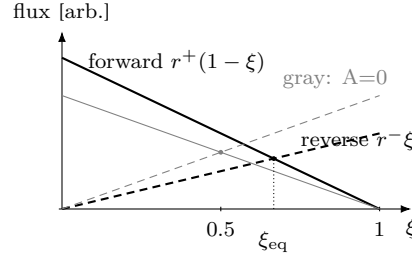
Figure 6: 정지점 유도 (신규). 정방향 플럭스 r^+(1 - \xi) (감소 직선)와 역방향 r^-\xi (증가 직선)의 교점이 정지점 \xi_{eq} (식 ??). \mathcal{A} > 0 ( r^+ = 2r^- , 검정)이면 \xi_{eq} = 2/3 , \mathcal{A} = 0 (회색)이면 \frac{1}{2} — detailed balance (식 ??)가 평형을 정한다.
