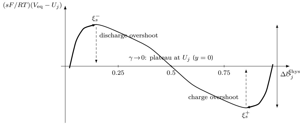
Figure 4: 비단조 평형 전위 V_{eq}(\xi) (식 (??), \Omega_j = 4RT )와 과주행(v7-11 유래). 방전(굵은 경로, 좌상)은 극대 \xi_s^- 까지, 충전(우하)은 극소 \xi_s^+ 까지 과주행해 중심이 갈라진다. 두 극값 차가 spinodal 상한 gap \Delta U_j^{hys} (식 (??)), 실측 분기는 \gamma_j 만큼 안쪽(식 (??)). \gamma \rightarrow 0 가역 한계에서 두 경로가 y = 0 plateau로 합쳐진다.
