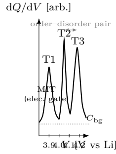
Figure 9: LCO 하프셀 dQ/dV 평형 peak 도식(신규, 정성). 세 종 = T1(MIT, \sim 3.90 V; 전자 게이트 구간이라 폭이 넓고 온도 민감), T2·T3(order-disorder 쌍, \sim 4.05/\sim 4.18 V). 각 봉우리는 같은 평형 종 Q_j \xi_{eq}(1 - \xi_{eq})/w_j (식 (1.43))이며 중심만 표 2로 바뀐다. 흑연(그림은 0.085–0.21 V)과 같은 forward 모델, 다른 전위 대. 전자 엔트로피는 T1 중심의 온도 이동에만 미세 기여한다.
