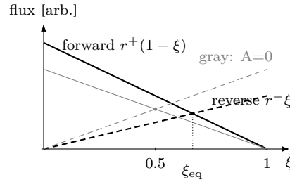
Figure 6: 정지점 유도(신규). 정방향 플럭스 r^+(1 - \xi) (감소 직선)와 역방향 r^-\xi (증가 직선)의 교점이 정지점 \xi_{eq} (식 (1.28)). \mathcal{A} > 0 ( r^+ = 2r^- , 검정)이면 \xi_{eq} = 2/3 , \mathcal{A} = 0 (회색)이면 \frac{1}{2} — detailed balance(식 (1.27))가 평형을 정한다.
