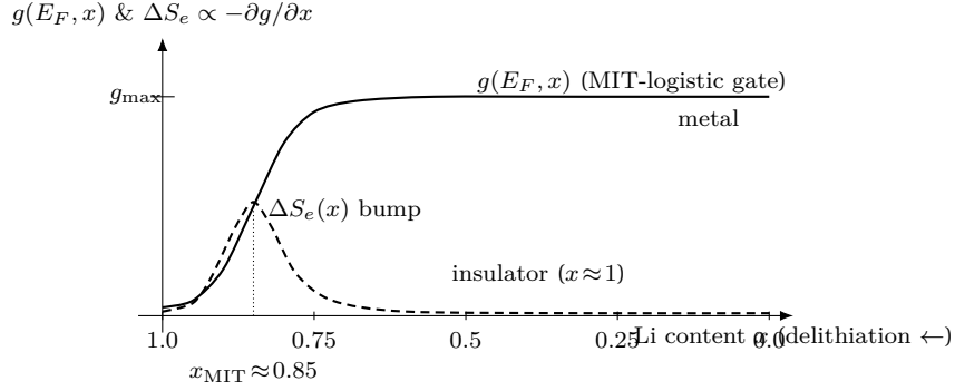
Figure 8: LCO 전자 엔트로피의 MIT-logistic 게이트(신규). 실선 = g(E_F, x) (식 (1.36)): x \approx 1 절연체에서 \approx 0 , 탈리튬화로 x_{MIT} \approx 0.85 부근에서 metal 의 g_{max} = 13 \text{ e/eV} 로 커진다. 파선 = 탈리튬화 시 방출되는 부분몰 전자 엔트로피 |\Delta S_e| = -\partial S_e / \partial x \propto -\partial g / \partial x > 0 (식 (1.34)·닫힌식 (1.37); 삽입 기준 \Delta S_e = \partial S_e / \partial x < 0 의 절댓값으로, x_{MIT} 에서 \sigma(1 - \sigma) 가 최대): 천이 중심의 국소 봉우리다 — 작지만(O3 부분몰 \approx 0.18 k_B/\text{atom} ) MIT 구간에만 커지는 게이트라 config 단독으로 대체 불가. \Delta S_{e,j} \propto T 라 다른 항과 달리 전자 기여의 \partial U / \partial T 가 T 에 선형 (§1.6.2; U-이동은 \propto T^2 ). 흑연엔 이 봉우리가 없다( g(E_F) 변화 미미).
