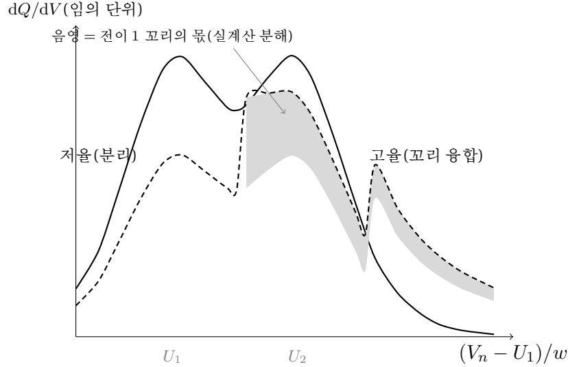
Figure 8: 두 인접 전이의 융합(중심 간격 3.9w ). 실선은 저울( r_a \rightarrow 0 ) — 골이 깊어 분리가 일어난다. 파선은 고울( r_a = 0.35 , L_V = 4w ) — 식 (1.68) 그대로, 중 향이 (1 - r_a) = 0.65 로 깎이고 각 전이의 꼬리가 다음 전이 쪽으로 뻗어 골의 우측을 매우고 뒤 어깨를 들어 올리므로 분리 판독이 지워진다. 음영 띠가 그 주변 — 고울 곡선에서 전이 1 꼬리가 보태는 뭉(실계산 분해: 진폭 r_a/L_V = 0.0875 의 지수) — 이며, 골 위와 전이 2의 어깨 위에 걸쳐 있는 것이 보인다. 저온도 같은 방향으로 작용한다.
