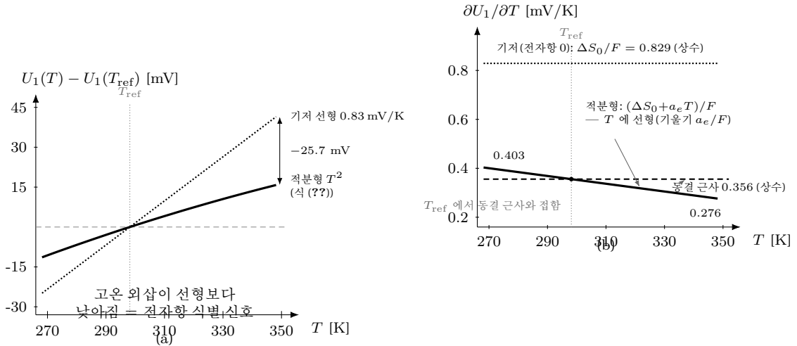
Figure 3: T1 전이 중심의 온도 함수형이 갖는 전자항 식별 신호 — 좌표는 식 (??) 그대로의 수치 평가다( \Delta S_0=+80 J/(mol K) 대표 스케일[tier B — §??], 게이트 중심의 몰당 단원식(식 (??)·(??)) 에서 a_e=-0.153 J/(mol K 2 ), T_{\text{ref}}=298.15 K). (a) U_1(T) : 전자항이 없으면 기저 선형(점선, 0.83 mV/K), 전자항( \propto T )을 적분하면 T^2 곡률(실선) — a_e < 0 라 고온 외삽이 선형 외삽보다 낮아지고 (348 K 에서 -25.7 mV) 이것이 다운도 피팅의 식별 신호다. (b) 같은 내용의 기울기 공간: \partial U_1 / \partial T = (\Delta S_0 + a_e T) / F 가 T 에 선형으로 감소한다( 0.403 \rightarrow 0.276 mV/K). 현행 동결 근사(파선 — \Delta S_e 를 T_{\text{ref}} 상수로 두는 §?? 의 단일-기준 근사)는 적분형의 T_{\text{ref}} 접선이라 (a)에서는 실선과 ( a_e/2F )( T - T_{\text{ref}} ) 2 (348 K 에서 -2.0 mV) 만큼만 이차로 벌어지고, (b)의 기울기 공간에서 상수 대 선형으로 명확히 갈린다.
