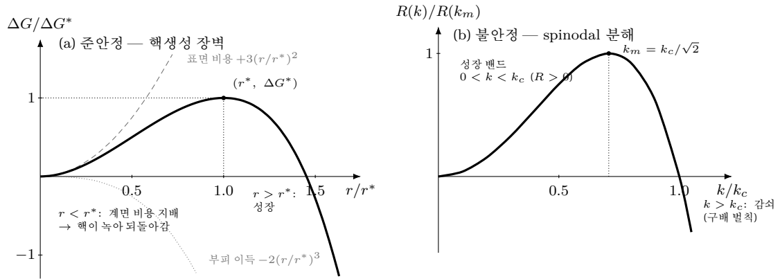
Figure 1: 준안정과 불안정 영역의 두 동역학 경로 — 좌표는 식 그대로의 수치 평가다. (a) 고전 핵생성: 구형 핵의 자유에너지 식 (??) 을 임계값 식 (??) 로 무차원화하면 \Delta G/\Delta G^* = 3(r/r^*)^2 - 2(r/r^*)^3 이다. 표면 비용( +r^2 , 파선)과 부피 이득( -r^3 , 점선)의 경쟁이 r^* 에서 장벽 \Delta G^* 를 만들고, r < r^* 인 핵은 되돌아가며 r > r^* 만 성장한다 — 준안정 영역의 분해가 \exp(-\Delta G^*/k_B T) 로 지수 억제되는 까닭이다. (b) spinodal 분해: 불안정 영역( f'' < 0 )의 모드별 성장률 식 (??) 을 최대 성장 모드로 무차원화하면 R(k)/R(k_m) = 4(k/k_c)^2[1 - (k/k_c)^2] 이며, 장벽 없이 0 < k < k_c 밴드 전체가 지수 성장하고 k_m = k_c/\sqrt{2} 물결이 가장 빨리 자란다. 장벽 유무가 두 영역(binodal-spinodal 사이 vs spinodal 안쪽)의 조작적 차이이다.
