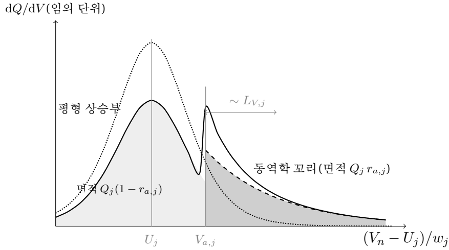
Figure 11: 단한식 (1.79) 한 전이의 해부( r_{a,j} = 0.315 , L_V = 3w ). 점선은 평형 중 (기준선), 파선은 동역학 꼬리, 실선이 단한식의 합이다. 상승부 실선이 점선보다 낮은 간격이 종 항의 (1 - r_{a,j}) 인자 — 꼬리로 넘어간 미완 몫의 회계 — 이고, 열은 음영(중 성분)과 진한 음영(꼬리 성분)의 면적이 각각 Q_j(1 - r_{a,j}) 와 Q_j r_{a,j} , 합이 정확히 Q_j 다(식 (1.80) 의 시각 짝). 꼬리는 V_{a,j} 에서 진폭 r_{a,j}/L_{V,j} 로 점화되어 단방향으로만 살며, 점화 계단은 지시함수의 모델 성질이라 r_{a,j} 가 클수록 크고 실측에서는 평활이 뭉갠다. 점화점 U_j + 2.25w 는 꼬리 형상이 한눈에 들어오도록 잡은 예시 배치다 — 실데이터의 V_{a,j} 는 컷 정의 (§1.15 (3'))가 그 조건의 측정 V_n(q) 위에서 정하며, 보통 종의 더 깊은 어깨에 맺힌다.
