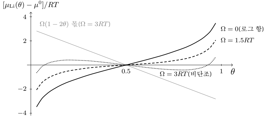
Figure 3: 화학퍼텐셜 (1.13)의 해부(실계산). 실선은 \Omega = 0 의 로그(섞임 엔트로피) 몫 — 채울수록 값어치가 단조로 오른다. 회색 가는 선은 상호작용 몫 \Omega(1-2\theta) ( \Omega = 3RT ) — 반대 기울기의 직선이다. 로그 몫에 각자의 \Omega(1-2\theta) 를 더하면: \Omega = 1.5RT (파선)는 가운데가 평평해진 단조 곡선, \Omega = 3RT > 2RT (점선)는 비단조 — 한 값어치에 세 조성이 대응하며, 이것이 상분리의 씨앗이다 (§1.5).
