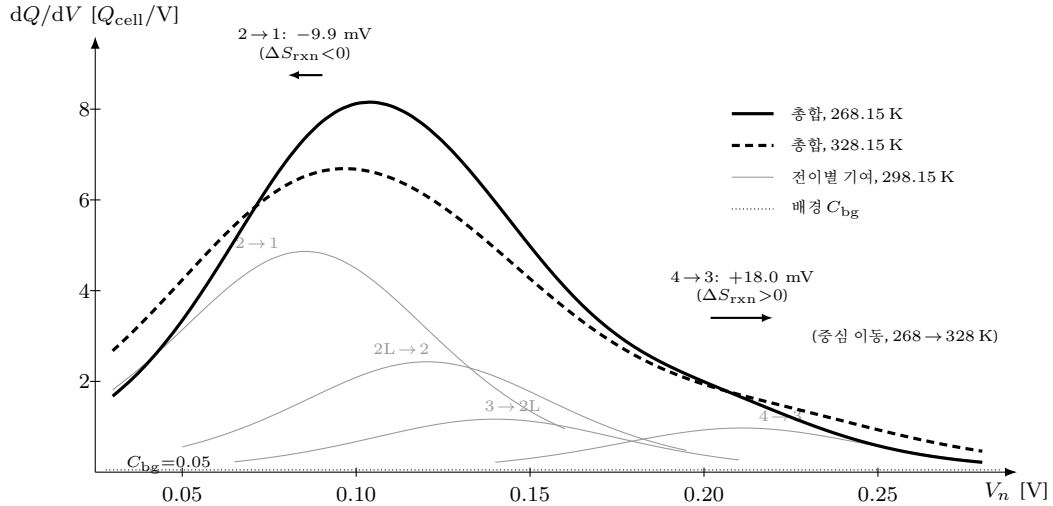
Figure 18: 합산식 (1.101) 이 내는 전체 곡선 — 좌표는 식 그대로의 수치 평가다: 초기 상태의 평형 중 전용 극한( L_V \rightarrow 0 \cdot \gamma_j = 0 \cdot R_n = 0 )에서 dQ/dV = C_{bg} + \sum_j Q_j \xi_{eq,j} (1 - \xi_{eq,j}) / w_j 를 표 2 초기값으로 평가했다( U_j(T) = (-\Delta H_{rxn,j} + T \Delta S_{rxn,j}) / F 를 온도마다 재평가, w_j = RT/F - n_j = 1 균일, 배경은 상수 예시 C_{bg} = 0.05 Q_{cell}/V ). 회색 가는 곡선이 298.15 K의 전이별 기여, 굵은 실선·파선이 268.15/328.15 K의 총합이다. 온도가 오르면 (i) 폭 w = RT/F 가 비례해 열려 봉우리가 낮고 넓어지고(면적 Q_j 보존), (ii) 중심은 \partial U_j / \partial T = \Delta S_{rxn,j} / F 를 따라 전이마다 반대 방향으로 움직인다 — 60 K 동안 2 \rightarrow 1 ( \Delta S_{rxn} = -16 \text{ J}/(\text{mol K}) )은 -9.9 \text{ mV} 로 왼쪽, 4 \rightarrow 3 (+29)은 +18.0 \text{ mV} 로 오른쪽(화살표), 3 \rightarrow 2L(0) 은 제자리다. 다운도 피팅에서 온도마다 U_j(T) 를 따로 읽어야 하는 까닭 (§1.3)이 이 한 장이다.
