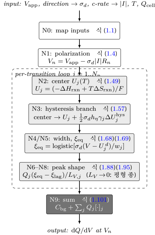
Figure 1: 한 곡선을 그리는 계산 진행(spine). 외부 실험조건 ( V_{\text{app}}, \text{direction}, c\text{-rate}, Q_{\text{cell}}, T ) 이 N0 에서 모델 입력 ( \sigma_d, |I| ) 로 환산되고(식 (1.1)), 분극으로 내부 전위 V_n 을 얻은 뒤(N1, 식 (1.4)), 과전 상자 안(전이별 반복 계산 단위, j = 1..N_p )에서 전이 j 마다 평형 중심(N2)·히스 분기(N3)·폭·평형 진행률(N4/N5)을 잇달아 계산하고, 자연 길이 L_V 와 peak 모양(N6-N8, 식 (1.88)·(1.95))을 단일 꼬리식으로 얻는다 — 평형 중(식 (1.75))은 그 L_V \rightarrow 0 극한이다(식 (1.99)). 모든 전이가 이 loop 를 마치면 N9(진한 상자, 식 (1.101))가 배경 위에 합산한다.
