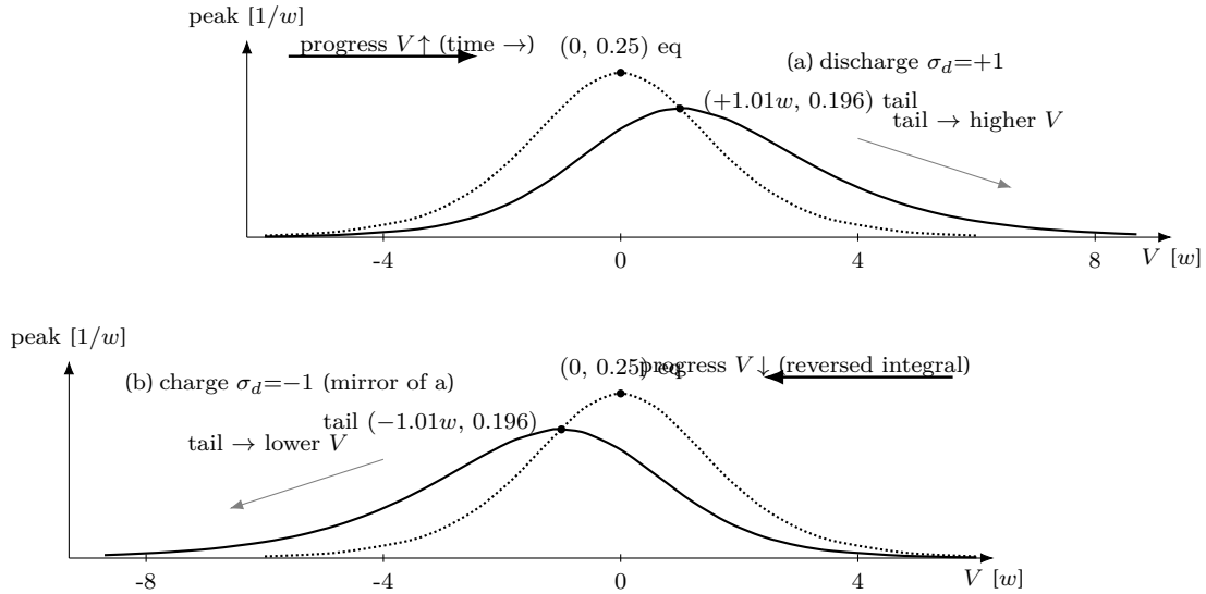
Figure 17: 인과 꼬리의 방향 — 좌표는 식 (1.94)·(1.100)의 점별 적분을 수치 평가한 값이다( w=1 , L_V=1.5w ). 점선 = 평형 중 \xi_{eq}(1 - \xi_{eq})/w (정점 0.25@중심, 방향 불변), 실선 = peak shape (\xi_{eq} - \xi_{lag})/L_V (식 (1.95)). (a) 방전은 진행이 V \uparrow 라 꼬리가 높은 V 쪽으로, 정점 (+1.01w, 0.196) (식 (1.100) 상단 분기). (b) 충전은 진행이 V \downarrow 라 인과 적분이 향하는 쪽이 뒤집혀(식 (1.100) 하단 분기) 꼬리가 낮은 V 쪽으로, 정점 (-1.01w, 0.196) — 방전의 정확한 거울. 두 경우 모두 peak 는 양수. (좌표는 기억 적분의 도식 수치평가다.)
