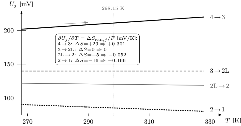
Figure 7: 평형 중심의 온도 의존 U_j(T) (식 (1.49); 좌표는 식 그대로의 수치 평가: 표 2의 네 전이 ( \Delta H_{\text{rxn},j} , \Delta S_{\text{rxn},j} ), T=268\text{--}328 K). 각 직선의 기울기가 정확히 \partial U_j/\partial T = \Delta S_{\text{rxn},j}/F 라, 반응 엔트로피의 부호가 중심의 이동 방향을 정한다 — \Delta S > 0 인 4 \rightarrow 3(+29) 은 온도가 오르면 중심이 올라가고, \Delta S = 0 인 3 \rightarrow 2L 은 평평하며, \Delta S < 0 인 2 \rightarrow 1(-16) · 2L \rightarrow 2(-5) 은 내려간다. 기울기 규모는 |\Delta S|/F \sim 수십 \mu\text{V/K} \sim 0.3 mV/K 이라 60 K 창에서 중심이 수~수십 mV 이동한다 — 다운도 피팅에서 온도마다 U_j(T) 를 따로 읽어야 하는 까닭이 이 서로 다른 기울기다. 세로축은 75 mV에서 끊어 그렸다.
