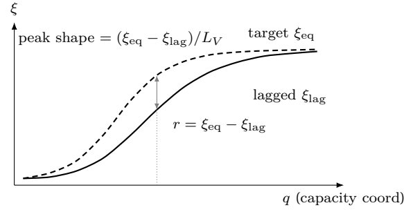
Figure 16: 지연의 완화. 파선 = 평형 목표 \xi_{eq}(q) , 실선 = 인과 기억 적분(식 (1.94))으로 뒤쳐진 \xi_{lag} . 둘의 차 r = \xi_{eq} - \xi_{lag} 가 지연이고, peak 모양 (\xi_{eq} - \xi_{lag})/L_V (식 (1.95))은 이 차를 길이로 나눈 것이다. L_{V,j} \rightarrow 0 에서 이 차분이 평형 종의 미분으로 매끈히 수렴하는 논증(식 (1.99))은 본문 §1.9 다음 소절이 다룬다. (좌표는 기억 적분의 도식 평가다.)
