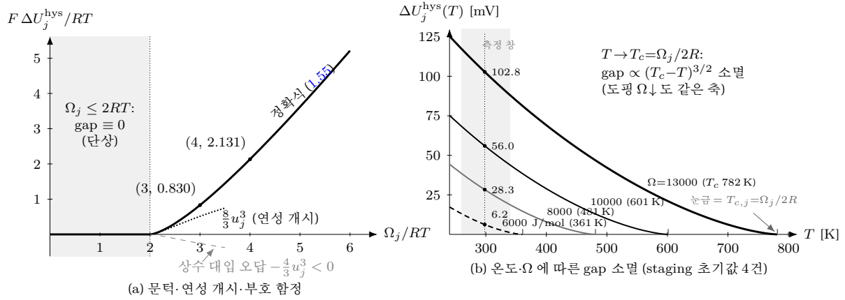
Figure 9: 히스테리시스 gap 닫힌 꼴 \Delta U_j^{\text{hys}} (식 (1.55))의 전 거동 — 좌표는 식 그대로의 수치 평가. (a) 무차원 gap F\Delta U_j^{\text{hys}}/RT = 2[\omega u_j - 2 \operatorname{artanh} u_j] ( \omega \equiv \Omega_j/RT , u_j = \sqrt{1 - 2/\omega} ): 문턱 \Omega_j \leq 2RT (음영)에서 정확히 0, 문턱 직후 두 급수를 함께 전개한 \frac{8}{3}u_j^3 (점선)으로 양수 연성 개시 하며, \Omega_j 를 상수 대입만 한 잘못된 전개는 -\frac{4}{3}u_j^3 (회색 파선)로 부호가 뒤집힌다(본문 ★Taylor 전개의 함정). 점 (4, 2.131)은 그림 10의 \Omega_j=4RT gap과 같은 값이다. (b) 표 2의 \Omega_j 초기값 4건을 mV로 평가한 \Delta U_j^{\text{hys}}(T) : 각 곡선은 자기 임계온도 T_{c,j} = \Omega_j/2R (축 눈금)에서 (T_c - T)^{3/2} 로 매끄럽게 소멸한다 — 승온과 도핑에 의한 \Omega_j 감소(식 (2.14))가 같은 축 위에서 gap을 닫는 두 조절 변수다. 점선 수직선은 298.15 K, 그 교점 수치는 spinodal 상한 gap이며 실측 분기는 \gamma_j 배 안쪽이다 (식 (1.57)).
