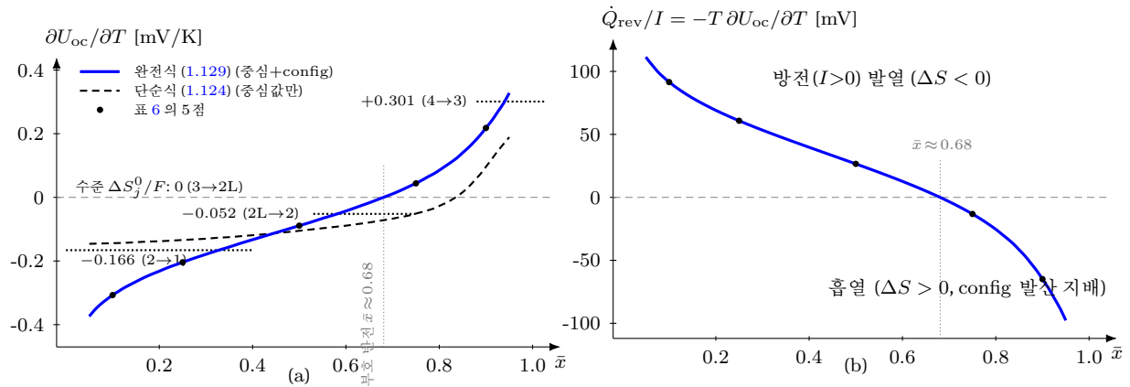
Figure 22: 완전식이 만드는 하프셀 엔트로피 계수와 가역 발열의 실제산 곡선 — 좌표는 식 그대로의 수치 평가다(4-전이 staging 입력: 표 3의 \Delta S_j^0 , w_j=RT/F(n_j=1) , 298.15 K; 각 \bar{x} 에서 전하 보존 음함수 (1.119)를 풀어 U_{oc} 를 얻은 뒤 평가). (a) \partial U_{oc}/\partial T(\bar{x}) — 파란 실선 = 완전식 (1.129)(중심 표준값+분포 config), 검은 파선 = 단순식 (1.124)(중심값만) 이고 둘의 차가 봉우리 내부 config 항이다(파생 B). 점선 수평선은 전이별 수준 \Delta S_j^0/F — 곡선이 전이 경계마다 계단 없이 인접 수준 사이를 연속으로 지난다(파생 A의 연속 블렌드). ●는 표 6의 다섯 점과 일치하며 \bar{x}=0.25 값이 계산 예제 (§1.18.2)의 -0.204/ 단순식 -0.134 mV/K 다. (b) 가역 발열 \dot{Q}_{rev}/I = -T \partial U_{oc}/\partial T (식 (1.128)) — \bar{x} \approx 0.68 에서 방전 발열이 흡열로 스스로 반전한다(임의 함수·외부 스위치 없이 분포만으로). 완전식 곡선은 폭의 열적 서식 w_j=n_jRT/F 를 전제하며, 실측 폭이 T -동결에 가까우면 단순식이 보수적 기준이다 (§1.15.4).
