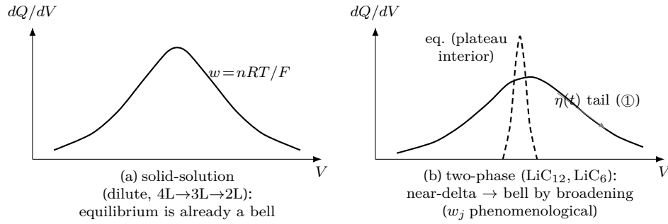
Figure 15: 평형 모양과 broadening. (a) 연속 고용체 전이 — 평형 단일 입자 dQ/dV 가 이미 폭 n_j RT/F 의 종(식 (1.75)), broadening 불요. (b) 두-상 전이 — 평형은 plateau 내부에서 거의 날카로운 선(파선; 양끝 단상 꼬리 탓에 폭이 정확히 0 은 아님)이고, 실측은 세 출처가 펼친 치우친 종(실선)이다: ① 유한율속 비대칭 꼬리 (§1.8–§1.9 의 L_V , |I| \rightarrow 0 소멸), ② 전류 무관한 가장자리 내재 폭 ( \sim RT/F ), ③ 겹보기 중심 U_{app} = U_j + \eta 의 입자간 \eta 산포를 forward 평균한 앙상블 뭉 (식 (1.76)). ①의 \eta(t) (한 입자의 시간 변화)와 ③의 입자간 \eta 산포는 같은 과전압의 다른 평균이며, 평형 중심 U_j 는 입자 무관 상수다 — 분포하는 것은 \eta . 세 출처의 지위와 한정(폭 w_j 의 현상학적 지위·흑연 두-상 국한· \rho(U_{app}) 역산 금지·사이즈 배제)은 본문 §1.7.2·§1.7.3.
