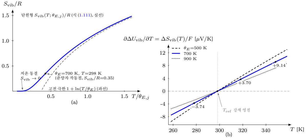
Figure 20: Einstein 진동 보정의 두 얼굴 — 좌표는 식 (1.111)·(1.113) 그대로의 수치 평가다. (a) 단진형 S_{\text{vib}}(T; \theta_{E,j})/R : 저온( u_j \rightarrow \infty )에서 0 으로 동결되고 고전 극한(파선) 1 + \ln(T/\theta_E) 에 T/\theta_E \gtrsim 1 에서 붙는다 — 앞 절이 중심 표준값에 흡수한 “ T -무관 상수”는 이 곡선을 T_{\text{ref}} 에서 한 번 평가해 동결한 값이다. ● 는 \theta_E = 700 \text{ K} · 298 \text{ K} 의 준양자 작동점. (b) 중심 이동의 온도 기울기 \partial \Delta U_{\text{vib}} / \partial T = \Delta S_{\text{vib}}(T)/F : \theta_E = 500/700/900 \text{ K} 모두 T_{\text{ref}} 의 강제 영점을 지나 로그형 곡률로 자라며, ● 는 본문 §1.14.3 의 수치 ( \theta_E = 700 \text{ K} 에서 -3.74/0/+3.70/+9.14 \mu\text{V/K} ) 다. electronic 항( \propto T )은 이 강제 영점이 없어 두 함수형이 다운도 곡률 피팅에서 갈리고, 분리에는 준양자 창을 걸치는 온도점 셋 이상이 필요하다.
