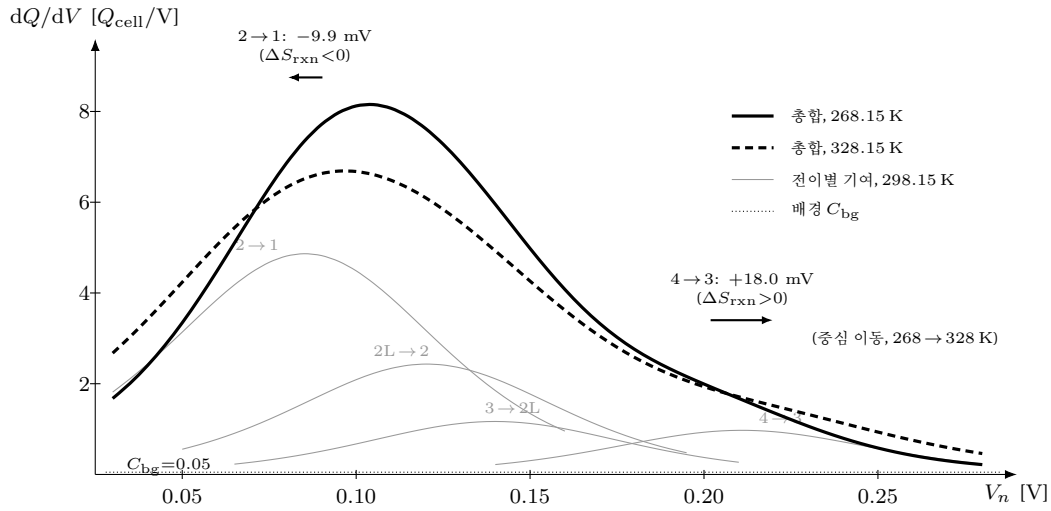
Figure 18: 합산식 (1.101) 이 내는 전체 곡선 — 좌표는 식 그대로의 수치 평가다: 초기 상태의 평형 중 전용 극한( L_V \rightarrow 0 \cdot \gamma_j = 0 \cdot R_n = 0 )에서 dQ/dV = C_{bg} + \sum_j Q_j \xi_{eq,j} (1 - \xi_{eq,j}) / w_j 를 표 2 초기값으로 평가했다( U_j(T) = (-\Delta H_{rxn,j} + T \Delta S_{rxn,j}) / F 를 온도마다 재평가, w_j = RT/F - n_j = 1 균일, 배경은 상수 예시 C_{bg} = 0.05 Q_{cell}/V ). 회색 가는 곡선이 298.15 K 의 전이별 기여, 굵은 실선·파선이 268.15/328.15 K 의 총합이다. 온도가 오르면 (i) 폭 w = RT/F 가 비례해 열려 봉우리가 낮고 넓어지고 (면적 Q_j 보존), (ii) 중심은 \partial U_j / \partial T = \Delta S_{rxn,j} / F 를 따라 전이마다 반대 방향으로 움직인다 — 60 K 동안 2 \rightarrow 1 ( \Delta S_{rxn} = -16 \text{ J}/(\text{mol K}) ) 은 -9.9 \text{ mV} 로 왼쪽, 4 \rightarrow 3 (+29) 은 +18.0 \text{ mV} 로 오른쪽(화살표), 3 \rightarrow 2L(0) 은 제자리다. 다운도 피팅에서 온도마다 U_j(T) 를 따로 읽어야 하는 까닭 (§1.3) 이 이 한 장이다.
