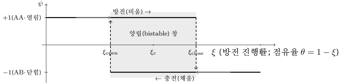
Figure 17: 적층 order parameter \psi 의 방향별 이력(식 (1.98)–(1.100); \xi_c = 0.5 , \Delta\xi_{\text{stack}} = 0.4 ). 충전 ( \xi 감소, 점유율 증가)은 닫힘( \psi = -1 )을 유지하다 \xi_{\text{open}} = 0.3 (점유율 70%)에서 열리고, 방전( \xi 증가)은 열림( \psi = +1 )을 \xi_{\text{close}} = 0.7 (점유율 30%)까지 버티다 닫는다(점선: 점화 점프; 가지는 \psi = \pm 1 로 이상화 — spinodal 부근 곡률은 생략). 두 임계 조성의 분리가 방향 비대칭이며, 음영의 bistable 창이 그 폭이다. B_j \rightarrow 0 에서 창이 닫혀 §1.13 의 대칭 그림으로 회수된다.
