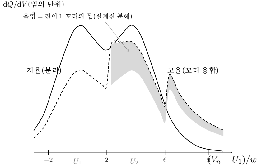
Figure 12: 두 인접 전이의 융합(중심 간격 3.9w ). 실선은 저울( r_a \rightarrow 0 ) — 골이 깊어 분리가 일어난다. 파선은 고울( r_a = 0.35 , L_V = 4w ) — 식 (1.82) 그대로, 중 항이 (1 - r_a) = 0.65 로 깎이고 각 전이의 꼬리가 다음 전이 쪽으로 뻗어 골의 우측을 매우고 뒤 어깨를 들어 올리므로 분리 판독이 지워진다. 음영 띠가 그 주변 — 고울 곡선에서 전이 1 꼬리가 보태는 뒤편(실계산 분해: 진폭 r_a/L_V = 0.0875 의 지수) —이며, 골 위와 전이 2의 어깨 위에 걸쳐 있는 것이 보인다. 저온도 같은 방향으로 작용한다.
