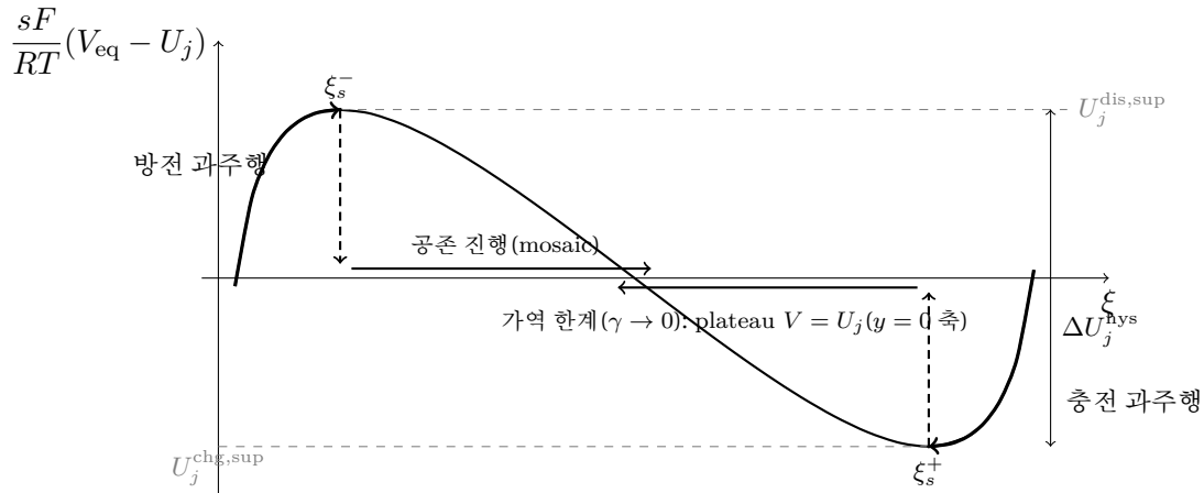
Figure 13: 비단조 평형 선위 (1.84)( \Omega_j = 4RT )와 과주행 경로 — 극값이 spinodal 에서는 근거는 식 (1.85). 방전(굵은 경로, 좌상)은 상승 준안정 가지를 타고 극대 \xi_s^- 까지 과주행한 뒤 분리가 점화된다 — 점선 화살표의 낙하는 점화된 입자 내부의 공존 완화이고, 집단의 운전 전위는 mosaic 전선이 분기 수준( U_j^{\text{dis}} 근방)에 붙들어 두므로 관측 plateau 가 y = 0 까지 내려오는 것은 \gamma \rightarrow 0 의 가역 한계에서다. 충전(우하)은 거울상으로 극소 \xi_s^+ 까지 과주행한다. 두 극값의 차가 spinodal 상한 gap \Delta U_j^{\text{hys}} 이고(위첨자 sup 는 spinodal 상한 표시), 실측 분기는 축소 인자 \gamma_j 만큼 그 안쪽에 선다 — \gamma \rightarrow 0 의 가역 한계에서 두 경로가 모두 y = 0 의 plateau 로 합쳐진다.
