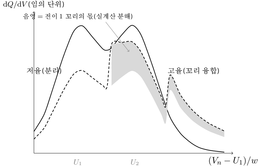
Figure 12: 두 인접 전이의 융합(중심 간격 3.9w ). 실선은 저울( r_a \rightarrow 0 ) — 골이 깊어 분리가 일어난다. 파선은 고울( r_a = 0.35, L_V = 4w ) — 식 (1.82) 그대로, 중 향이 (1 - r_a) = 0.65 로 깎이고 각 전이의 꼬리가 다음 전이 쪽으로 뻗어 골의 우측을 매우고 뒤 어깨를 들어 올리므로 분리 판독이 지워진다. 음영 띠가 그 주변 — 고울 곡선에서 전이 1 꼬리가 보태는 뭉(실계산 분해: 진폭 r_a/L_V = 0.0875 의 지수) — 이며, 골 위와 전이 2 의 어깨 위에 걸쳐 있는 것이 보인다. 저온도 같은 방향으로 작용한다.
