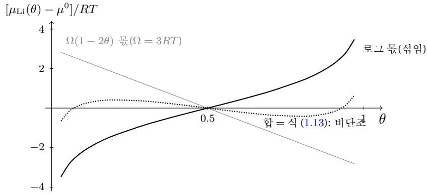
Figure 3: 화학퍼텐셜 (1.13) 한 곡선의 분해(실계산, \Omega = 3RT ). 실선은 로그(섞임 엔트로피) 몫 — 채울수록 값어치가 단조로 오른다. 회색 직선은 상호작용 몫 \Omega(1 - 2\theta) — 반대 기울기다. 둘의 합(점선)이 식 (1.13) 그 자체이고, \Omega > 2RT 라 비단조 — 한 값어치에 세 조성이 대응하며 이것이 상분리의 씨앗이다 (§1.5). \Omega 를 바꿔 가며 본 가족 비교는 전위축의 등온선 그림 5 이 말한다 — 두 그림은 같은 식의 다른 두 절단이다.
