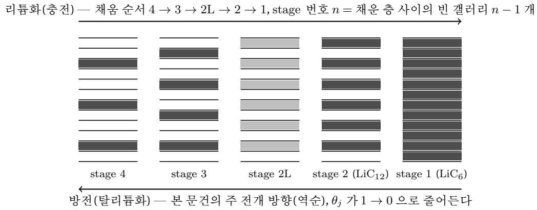
Figure 1: 흑연 staging의 갤러리 채움 도식. 수평선이 그려진 층, 음영 띠가 리튬이 든 층간 갤러리다. 채울수록 stage 번호가 줄어 stage 1(LiC 6 , 완전 채움)에 닿고, 각 stage 전이가 dQ/dV 에 peak 하나를 남긴다. stage 2L 은 stage 2 와 같은 주기이되 갤러리 안이 희박하고 면내 질서가 풀린(liquid-like) 단계라 열게 표시했다. 개념도이며 — 실제 채움은 갤러리 전체가 아니라 국소 도메인 단위로 진행되고 층의 굽힘을 동반한다(Daumas-Hérolld 그림, §1.3).
