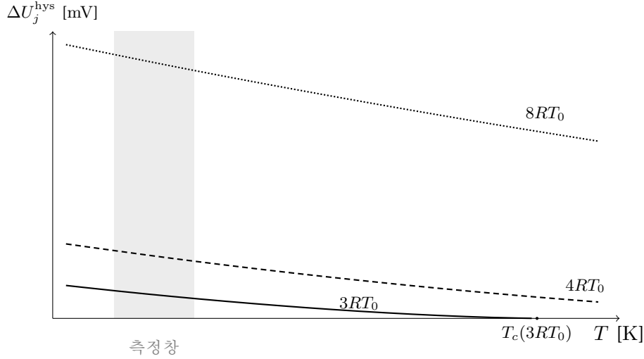
Figure 9: spinodal gap \Delta U_j^{\text{hys}}(T) (식 (1.57)), \Omega_j = 3/4/8RT_0 . 음영이 측정창(15–45°C)이다. T_{c,j} 가 창에 가까울수록 창 안의 감소가 가팔라 \Omega_j 식별이 잘 되고, 깊은 2상측은 거의 평탄해 퇴화 처리가 필요하다. T \rightarrow T_{c,j} 에서 (T_c - T)^{3/2} 맥으로 소멸한다.
