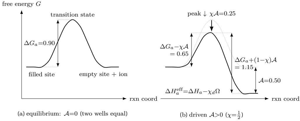
Figure 9: 활성화 장벽 그림 — Eyring 속도식(식 (1.50))의 반응 좌표 개형(좌표는 모형 이중웰 퍼텐셜 G_{\text{base}} = 0.1 + 0.9 \sin^2[\pi(x-1)/4] 의 수치 평가, 구동은 진행률 \phi 를 따라 A 만큼 기울임). (a) 평형( A=0 ) — 두 골 같은 높이, 장벽 \Delta G_a = 0.90 . (b) 구동력 \mathcal{A}_j = sF(V_n - U_j) > 0 ( \chi = \frac{1}{2} )가 도착 골을 A=0.50 내려 정점을 \chi A = 0.25 낮추면, 정방향 장벽 \Delta G_a - \chi A = 0.65 로 하강·역방향 \Delta G_a + (1-\chi)A = 1.15 로 상승(점선=(a)). \chi \cdot (1-\chi) 분할이 detailed balance(식 (1.51))를 강제하고, 유효 장벽은 \Delta H_a^{\text{eff}} = \Delta H_a - \chi_d \Omega 다. 이 그림이 logistic(식 (1.54))과 L_q 의 공통 출발점이다.
