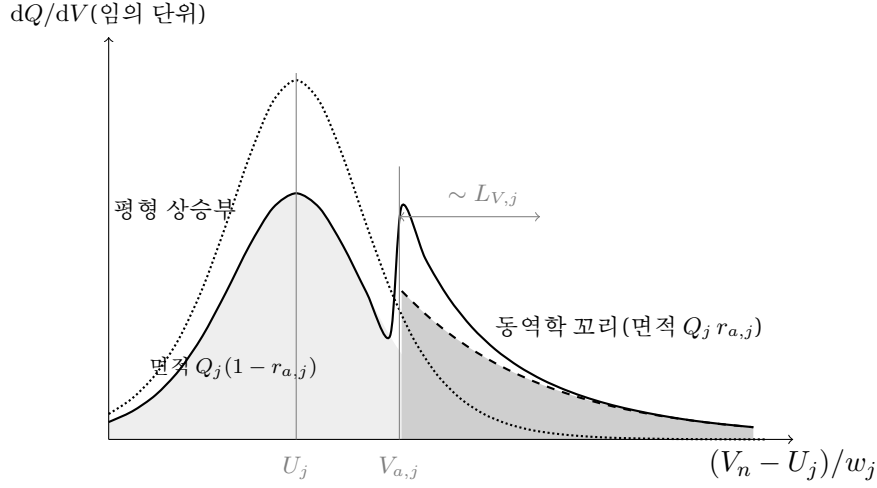
Figure 7: 닫힌식 (1.71) 한 전이의 해부( r_{a,j} = 0.315 , L_V = 3w ). 점선은 평형 종(기준선), 파선은 동역학 꼬리, 실선이 닫힌식의 합이다. 상승부 실선이 점선보다 낮은 간격이 종 항의 (1 - r_{a,j}) 인자 — 꼬리로 넘어간 미완 몫의 회계 — 이고, 열은 음영(종 성분)과 진한 음영(꼬리 성분)의 면적이 각각 Q_j(1 - r_{a,j}) 와 Q_j r_{a,j} , 합이 정확히 Q_j 다(식 (1.72)의 시각 짝). 꼬리는 V_{a,j} 에서 진폭 r_{a,j}/L_{V,j} 로 점화되어 단방향으로만 살며, 점화 계단은 지시함수의 모델 성질이라 r_{a,j} 가 클수록 크고 실측에서는 평활이 뭉갸다. 점화점이 U_j + 2.2w 에 놓인 것은 본 그림의 합성 조건에서 q -축 5% 컷이 맞히는 V -축 상(像)이라서다 — |dV/dq| 압축 때문에 V -축의 평형 종은 그 점에서 아직 유한하다.
