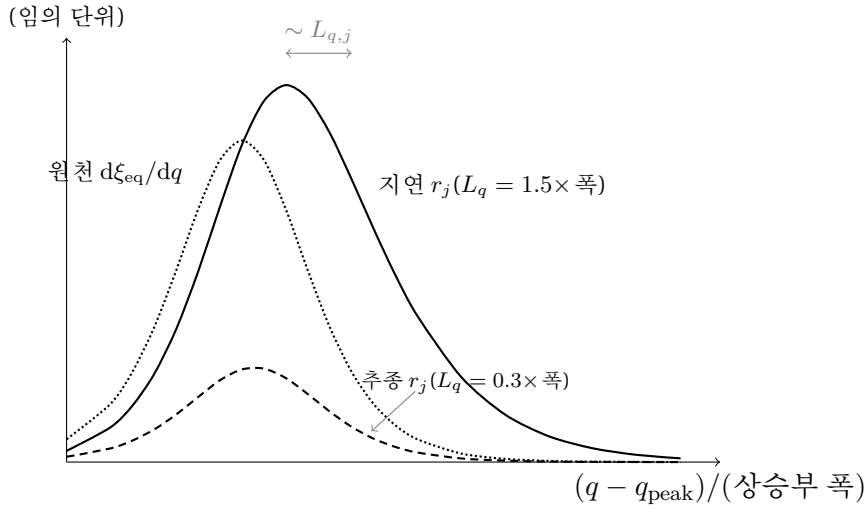
Figure 5: 일반해의 기억 거동(실계산, 두 케이스). 점선은 원천(평형 목표의 변화율). 파선은 L_q = 0.3 \times 상승부 폭 — 지연이 식 (1.54) 그대로 L_q d\xi_{eq}/dq 로 원천을 축소 추종하고(정점 높이 \approx L_q \times 원천 정점), 정점 이동도 커널 평균 \sim L_q (§1.11에서 정량)에 머문다. 실선은 L_q = 1.5 \times 폭 — 기억이 상승부를 통째로 덮어 정점이 원천보다 낮고 높으며, 원천이 포화로 꺼진 뒤에는 식 (1.55)의 순수 지수 감쇠로 넘어간다. 상승부 극한(추종)과 꼬리 극한(지수 기억)이 같은 일반해 (1.52)의 두 얼굴임을 한 그림으로 보였다(인용한 두 극한 식은 바로 다음 소절에서 유도된다).
