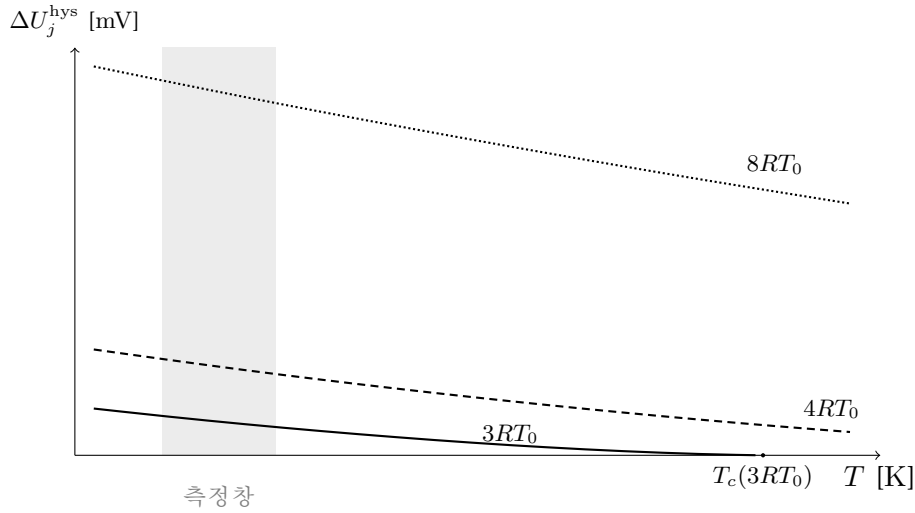
Figure 9: spinodal gap \Delta U_j^{\text{hys}}(T) (식 (1.58)), \Omega_j = 3/4/8RT_0 . 음영이 측정창(15–45°C)이다. T_{c,j} 가 창에 가까울수록 창 안의 감소가 가팔라 \Omega_j 식별이 잘 되고, 깊은 2상측은 거의 평탄해 퇴화 처리가 필요하다. T \rightarrow T_{c,j} 에서 (T_c - T)^{3/2} 먹으로 소멸한다.
