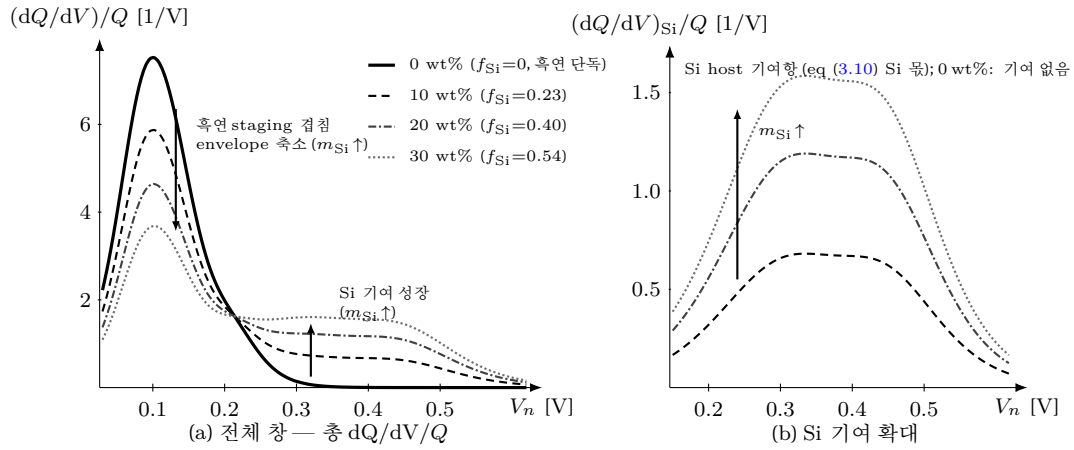
Figure 2: 블렌드 f_{Si} (wt% 스위치) 가족 평형 dQ/dV — 좌표는 코드 BlendedAnodeDQDV.from_wt( m_{Si} , si\_case='elemental' ) 의 실제산이다: 평형식 (3.10)의 |I| \rightarrow 0 중 \sum_{host} \sum_j Q_j^{host} \xi_{eq,j}^{host} (1 - \xi_{eq,j}^{host}) / w_j^{host} 을 T=298.15 K· C_{bg}=0 에서 평가하고 총용량 Q=Q_{gr}+Q_{Si} 로 정규화했다(곡선 아래 면적 = 1 규약, 곡선당 ~53–66 표본점). 질량↔용량 환산은 §3.3.1 각주의 환산 규약 f_{Si} = m_{Si}q_{Si} / [m_{Si}q_{Si} + (1-m_{Si})q_{gr}] ( q_{Si}=1000 mAh/g 원소 Si 1차 가역[2], tier-A· q_{gr}=372 )로, m_{Si}=0/10/20/30 wt% \Rightarrow f_{Si}=0/0.230/0.402/0.535 ( Q=0.97/1.26/1.62/2.09 Q_{cell} ). (a) 전체 창: 흑연 staging 4-peak 겹침 envelope는 m_{Si} 증가로 정규화 높이가 7.5 \rightarrow 3.7 [1/V]로 축소하고( Q_{gr} 절대값은 불변이나 총용량 Q 가 커져 상대 몫 1-f_{Si} 로 줄어듦), 원소 Si 두 경사 전이(중심 0.30/0.45 V, 폭 0.060/0.050 V)의 기여가 고전위 쪽에서 성장해 V_n \approx 0.26 V 부근에서 순서가 역전한다. (b) 그 Si host 몫만 떼어(코드 host_contributions ) 확대: 0 \rightarrow 1.585 [1/V]로 자란다( f_{Si} 에 정비례). 곡선 개형(전이 중심·폭)은 원소 Si 평균 전위대 0.2–0.5 V[10](tier-B)안의 tier-C 시연값이며(신뢰값 아님, 피팅 override 전제), elemental 케이스는 SiO_x 절대전위 같은 “확인 필요” 공백을 쓰지 않는다. f_{Si} \rightarrow 0 에서 (a)의 실선은 흑연 단독 평형곡선과 부동소수점까지 일치한다(bit-exact, 식 (3.9)의 코드판; §1.10 그림 18와 동일 흑연 골격).
