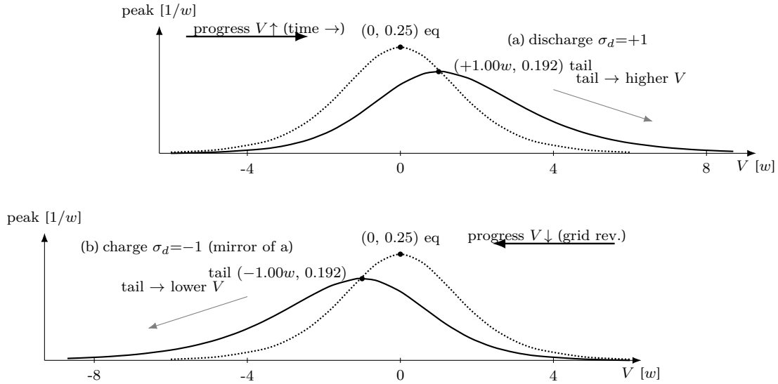
Figure 15: 인과 꼬리의 방향 — 좌표는 저역통과 점화식(식 (1.73))의 수치 평가( w=1 , L_V=1.5w , \rho=e^{-\Delta_{\text{grid}}/L_V}=0.967 ). 점선 = 평형 중 \xi_{\text{eq}}(1-\xi_{\text{eq}})/w (정점 0.25@중심, 방향 불변), 실선 = peak shape ( (\xi_{\text{eq}}-\xi_{\text{lag}})/L_V (식 (1.74))). (a) 방전은 진행이 V\uparrow 라 꼬리가 높은 V 쪽으로, 정점 (+1.00w, 0.192) (격자 그대로). (b) 충전은 진행이 V\downarrow 라 격자를 뒤집어 필터한 뒤 되돌려(식 (1.76)) 꼬리가 낮은 V 쪽으로, 정점 (-1.00w, 0.192) — 방전의 정확한 거울. 두 경우 모두 peak 는 양수.
