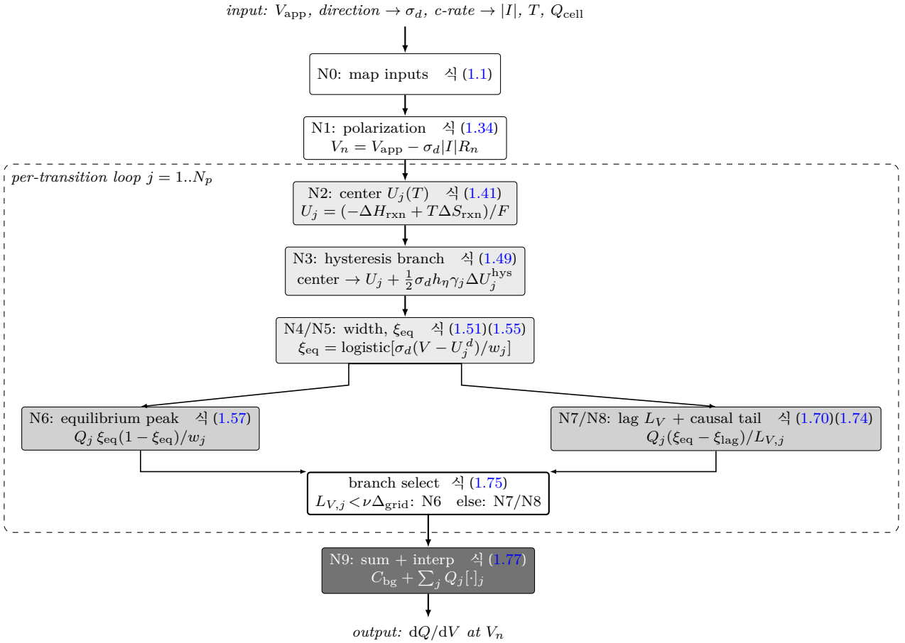
Figure 1: 한 곡선을 그리는 계산 진행(spine). 외부 실험조건 ( \sigma_d, |I|, T, Q_{cell} ) 이 N0 에서 모델 입력으로 환산되고(식 (1.1)), 분극으로 내부 전위 V_n 을 얻은 뒤(N1, 식 (1.34)), 파선 상자 안(전이별 반복 계산 단위, j = 1..N_p )에서 전이 j 마다 평형 중심(N2)·히스 분기(N3)·폭·평형 진행률(N4/N5)을 잇달아 계산한다. 열은 회색 상자 둘(N6 vs N7/N8)은 그 뒤 갈리는 두 경로다 — 식 (1.75)의 문턱 L_{V,j} < \nu\Delta_{grid} 이 평형 종(N6, 식 (1.57))과 지연 꼬리(N7/N8, 식 (1.70)·(1.74)) 중 하나를 고르는 분기 선택(굵은 테두리 상자)으로 합류한다. 모든 전이가 이 loop 를 마치면 N9(진한 상자, 식 (1.77))가 배경과 합산·역보간한다.
