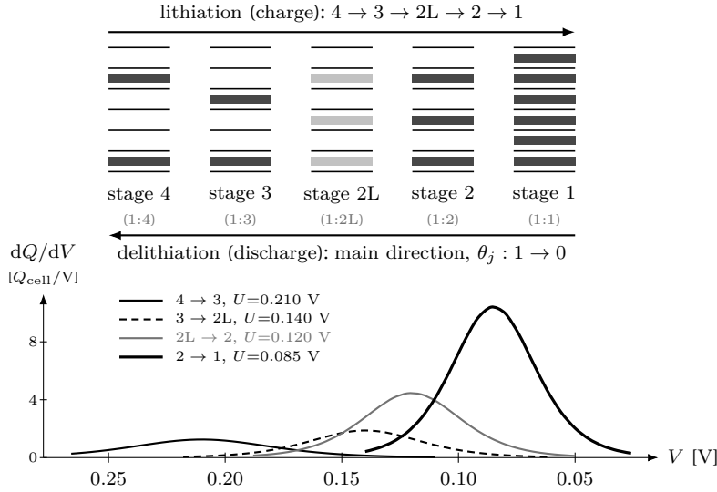
Figure 2: 흑연 staging의 갤러리 채움 도식(위)과 대응 dQ/dV peak(아래, 식 (1.57)의 초기값 수치 평가 — dQ/dV = Q_j \xi_{eq}(1 - \xi_{eq})/w_j , 표 2의 U_j, Q_j, w_j ). 위: 수평선이 그려진 층, 음영 띠가 리튬이 든 층간 갤러리다. 채울수록 stage 번호가 줄어 stage 1(LiC 6 , 완전 채움)에 닿고, 열 아래 비율(1:4→1:1)이 각 stage의 갤러리 점유 주기다. stage 2L은 면내 질서가 풀린 단계라 열게 표시했다. 아래: 네 초기값 전이의 실제 peak — 높이 Q_j/(4w_j) 는 전이마다 크게 다르다 ( 2 \rightarrow 1 이 가장 큼, 10.4 Q_{cell}/V ). 주의 — 위 갤러리 열 간격은 범주형(등간격 스케치)이고 아래 V 축은 실제 전위 스케일(비등간격 — 3 \rightarrow 2L 과 2L \rightarrow 2 은 겨우 20 mV 차이로 갤러리 열 간격에 선형 정렬되지 않는다)이라, 둘은 전이명(예 2 \rightarrow 1 )으로만 대응시킨다. 본 문건 방향은 방전(탈리튬화)이다.
