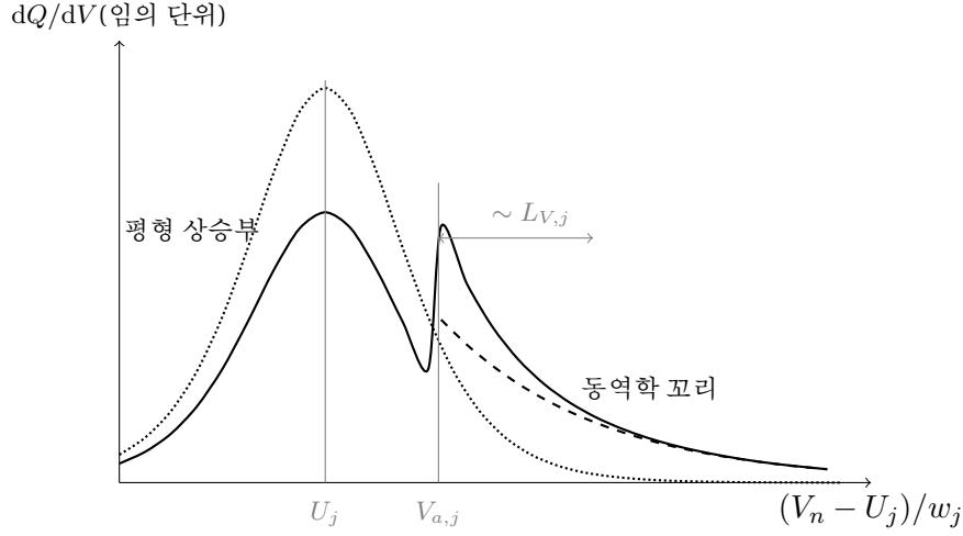
Figure 6: 닫힌식 (1.46) 한 전이의 해부( r_{a,j} = 0.315 , L_V = 3w ). 점선은 평형 중 (기준선), 파선은 동역학 꼬리, 실선이 닫힌식의 합이다. 상승부 실선이 점선보다 낮은 간격이 종 항의 (1 - r_{a,j}) 인자 — 꼬리로 넘어간 미완 몫의 회계 — 다. 꼬리는 V_{a,j} 에서 진폭 r_{a,j}/L_{V,j} 로 점화되어 단방향으로만 살며, 점화 계단은 지시함수의 모델 성질이라 r_{a,j} 가 클수록 크고 실측에서는 평활이 뭉갸다. 점화점이 U_j + 2.2w 에 놓인 것은 본 그림의 합성 조건에서 q -축 5% 컷이 맺히는 V -축 상(像)이라서다 — |dV/dq| 압축 때문에 V -축의 평형 중은 그 점에서 아직 유한하다.
