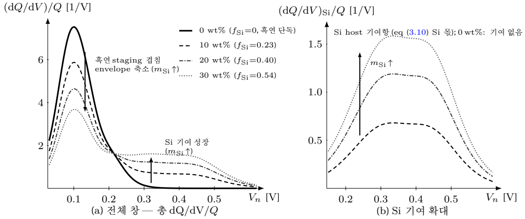
Figure 2: 블렌드 f_{\text{Si}} (wt% 스왑) 가족 평형 dQ/dV — 좌표는 원소 Si(elemental) host 블렌드의 평형 식 (3.10) 실제산이다: 그 |I| \rightarrow 0 중 \sum_{\text{host}} \sum_j Q_j^{\text{host}} \xi_{\text{eq},j}^{\text{host}} (1 - \xi_{\text{eq},j}^{\text{host}}) / w_j^{\text{host}} 을 T=298.15 \text{ K} \cdot C_{\text{bg}}=0 에서 평가하고 총용량 Q=Q_{\text{gr}}+Q_{\text{Si}} 로 정규화했다(곡선 아래 면적 = 1 규약, 곡선당 ~53–66 표본점). 질량↔용량 환산은 §3.3.1 각주의 환산 규약 f_{\text{Si}} = m_{\text{Si}}q_{\text{Si}} / [m_{\text{Si}}q_{\text{Si}} + (1-m_{\text{Si}})q_{\text{gr}}] ( q_{\text{Si}}=1000 \text{ mAh/g} 원소 Si 1차 가역[2], tier-A· q_{\text{gr}}=372 )로, m_{\text{Si}}=0/10/20/30 \text{ wt\%} \Rightarrow f_{\text{Si}}=0/0.230/0.402/0.535 ( Q=0.97/1.26/1.62/2.09 Q_{\text{cell}} ). (a) 전체 창: 흑연 staging 4-peak 겹침 envelope 는 m_{\text{Si}} 증가로 정규화 높이가 7.5 → 3.7 [1/V] 로 축소하고( Q_{\text{gr}} 절대값은 불변이나 총용량 Q 가 커져 상대 몫 1-f_{\text{Si}} 로 줄어듦), 원소 Si 두 경사 전이(중심 0.30/0.45 V, 폭 0.060/0.050 V)의 기여가 고전위 쪽에서 성장해 V_n \approx 0.26 \text{ V} 부근에서 순서가 역전한다. (b) 그 Si host 몫만 떼어 확대: 0 → 1.585 [1/V] 로 자란다( f_{\text{Si}} 에 정비례). 곡선 개형(전이 중심·폭)은 원소 Si 평균 전위대 0.2–0.5 V[10](tier-B) 안의 tier-C 시연값이며(신뢰값 아님, 피팅 override 전제), 원소 Si(elemental) 케이스는 \text{SiO}_x 절대전위 같은 “확인 필요” 공백을 쓰지 않는다. f_{\text{Si}} \rightarrow 0 에서 (a)의 실선은 흑연 단독 평형곡선과 부동소수점까지 일치한다(bit-exact, 식 (3.9)); §1.10 그림 18 와 동일 흑연 골격).
