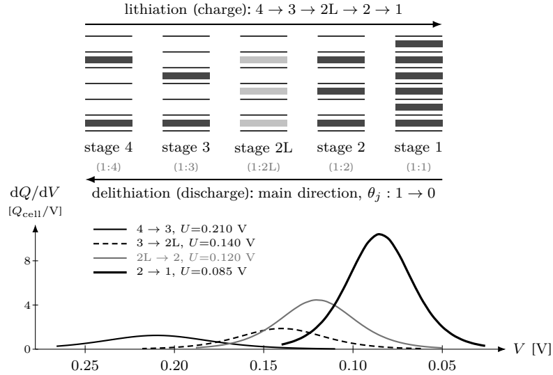
Figure 2: 흑연 staging 의 갤러리 채움 도식(위)과 대응 dQ/dV peak(아래, 식 (1.76) 의 수치 평가 — dQ/dV = Q_j \xi_{\text{eq}}(1 - \xi_{\text{eq}})/w_j , 표 2 의 U_j, Q_j 와 §1.10 폭 폴백 w_j ). 위: 수평선이 그려진 층, 음영 띠가 리튬이 든 층간 갤러리다. 채울수록 stage 번호가 줄어 stage 1( \text{LiC}_6 , 완전 채움)에 닿고, 열 아래 비율(1:4→1:1)이 각 stage 의 갤러리 점유 주기다. stage 2L 은 먼내 질서가 풀린 단계라 열게 표시했다. 아래: 폭 폴백 값으로 평가한 네 전이 peak — 높이 Q_j/(4w_j) 는 전이마다 크게 다르다 ( 2 \rightarrow 1 이 가장 큼, 10.4 Q_{\text{cell}}/V ; n_j=1 우선의 실제 초기 폭 w=RT/F 에서는 4.87 — §1.10). 주의 — 위 갤러리 열 간격은 범주형(등간격 스케치)이고 아래 V 축은 실제 전위 스케일(비등간격 — 3 \rightarrow 2L 과 2L \rightarrow 2 은 겨우 20 mV 차이로 갤러리 열 간격에 선형 정렬되지 않는다)이라, 둘은 전이명(예 2 \rightarrow 1 )으로만 대응시킨다. 본 장 방향은 방전(탈리튬화)이다.
