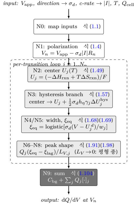
Figure 1: 한 곡선을 그리는 계산 진행(spine). 외부 실험조건 ( V_{app}, direction, c\_rate, Q_{cell}, T ) 이 N0 에서 모델 입력 ( \sigma_d, |I| ) 로 환산되고(식 (1.1)), 분극으로 내부 전위 V_n 을 얻은 뒤(N1, 식 (1.4)), 과전 상자 안(전이별 반복 계산 단위, j = 1..N_p )에서 전이 j 마다 평형 중심(N2)·히스 분기(N3)·폭·평형 진행률(N4/N5)을 잇달아 계산하고, 자연 길이 L_V 와 peak 모양(N6-N8, 식 (1.91)·(1.98))을 단일 꼬리식으로 얻는다 — 평형 중(식 (1.76))은 그 L_V \rightarrow 0 극한이다(식 (1.102)). 모든 전이가 이 loop 를 마치면 N9(진한 상자, 식 (1.104))가 배경 위에 합산한다.
