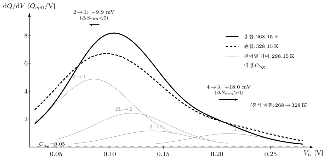
Figure 18: 합산식 (1.104) 이 내는 전체 곡선 — 좌표는 식 그대로의 수치 평가다: 초기 상태의 평형 중 전용 극한( L_V \rightarrow 0 \cdot \gamma_j = 0 \cdot R_n = 0 )에서 dQ/dV = C_{bg} + \sum_j Q_j \xi_{eq,j} (1 - \xi_{eq,j}) / w_j 를 표 2 초기값으로 평가했다( U_j(T) = (-\Delta H_{rxn,j} + T\Delta S_{rxn,j})/F 를 온도마다 재평가, w_j = RT/F - n_j = 1 균일, 배경은 상수 예시 C_{bg} = 0.05 Q_{cell}/V ). 회색 가는 곡선이 298.15 K의 전이별 기여, 굵은 실선·파선이 268.15/328.15 K의 총합이다. 온도가 오르면 (i) 폭 w = RT/F 가 비례해 열려 봉우리가 낮고 넓어지고 (면적 Q_j 보존), (ii) 중심은 \partial U_j / \partial T = \Delta S_{rxn,j} / F 를 따라 전이마다 반대 방향으로 움직인다 — 60 K 동안 2 \rightarrow 1 ( \Delta S_{rxn} = -16 \text{ J}/(\text{mol K}) )은 -9.9 \text{ mV} 로 왼쪽, 4 \rightarrow 3 (+29)은 +18.0 \text{ mV} 로 오른쪽(화살표), 3 \rightarrow 2L(0) 은 제자리다. 다운도 피팅에서 온도마다 U_j(T) 를 따로 읽어야 하는 까닭 (§1.3)이 이 한 장이다.
