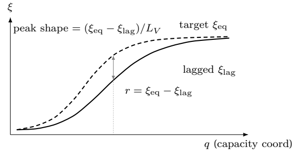
Figure 16: 지연의 완화. 파선 = 평형 목표 \xi_{eq}(q) , 실선 = 인과 기억 적분(식 (1.97))으로 뒤쳐진 \xi_{lag} . 둘의 차 r = \xi_{eq} - \xi_{lag} 가 지연이고, peak 모양 (\xi_{eq} - \xi_{lag})/L_V (식 (1.98))은 이 차를 길이로 나눈 것이다. L_{V,j} \rightarrow 0 에서 이 차이가 평형 중의 미분으로 매끈히 수렴하는 논증(식 (1.102))은 본문 §1.9 다음 소절이 닫는다. (좌표는 기억 적분의 도식 평가다.)
