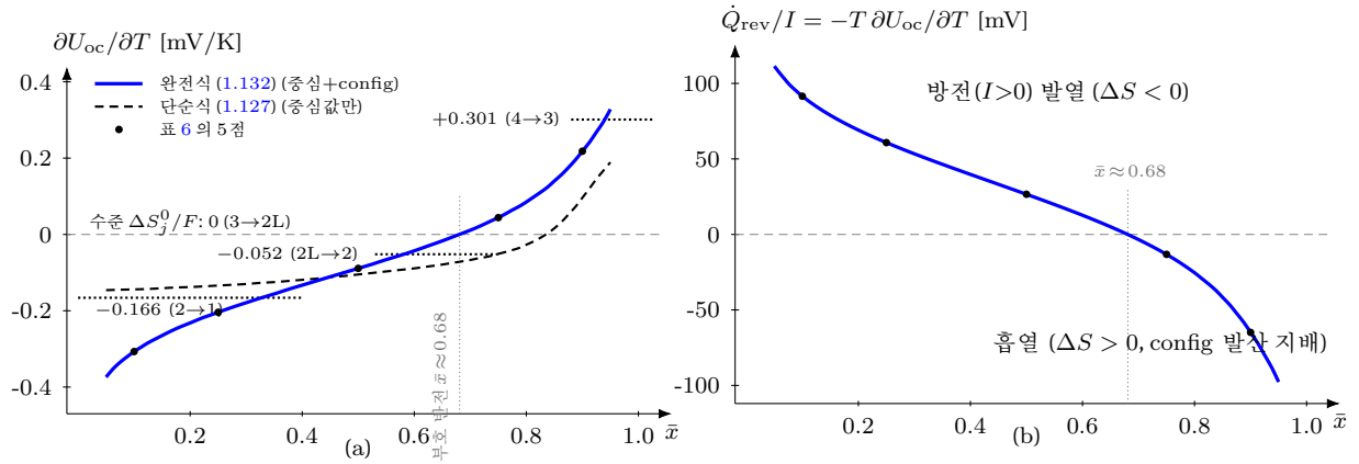
Figure 22: 완전식이 만드는 하프셀 엔트로피 계수와 가역 발열의 실제산 곡선 — 좌표는 식 그대로의 수치 평가다(4-전이 staging 입력: 표 3의 \Delta S_j^0 , w_j=RT/F(n_j=1) , 298.15 K; 각 \bar{x} 에서 전하 보존 음함수 (1.122)를 풀어 U_{oc} 를 얻은 뒤 평가). (a) \partial U_{oc}/\partial T(\bar{x}) — 파란 실선 = 완전식 (1.132)(중심 표준값+분포 config), 검은 파선 = 단순식 (1.127)(중심값만) 이고 둘의 차가 봉우리 내부 config 항이다(파생 B). 점선 수평선은 전이별 수준 \Delta S_j^0/F — 곡선이 전이 경계마다 계단 없이 인접 수준 사이를 연속으로 지난다(파생 A의 연속 블렌드). ●는 표 6의 다섯 점과 일치하며 \bar{x}=0.25 값이 계산 예제 (§1.18.2)의 -0.204/ 단순식 -0.134 mV/K 다. (b) 가역 발열 \dot{Q}_{rev}/I = -T\partial U_{oc}/\partial T (식 (1.131)) — \bar{x} \approx 0.68 에서 방전 발열이 흡열로 스스로 반전한다(임의 함수·외부 스위치 없이 분포만으로). 완전식 곡선은 폭의 열적 서식 w_j=n_jRT/F 를 전제하며, 실측 폭이 T -동결에 가까우면 단순식이 보수적 기준이다 (§1.15.4).
