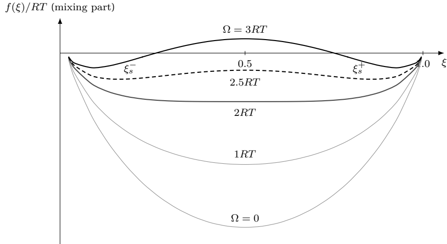
Figure 4: 정규용액 조성 자유에너지의 섞임 몫 f(\xi)/RT = \xi \ln \xi + (1-\xi) \ln(1-\xi) + (\Omega/RT) \xi(1-\xi) (좌표는 식 그대로의 수치 평가). \Omega < 2RT 면 한 웰, \Omega = 2RT 에서 바닥이 평탄해지고 (문턱, 식 (1.31)), \Omega > 2RT 면 가운데가 언덕이 된 이중웰 — \Omega = 3RT 곡선의 점이 spinodal \xi_s^\pm = 0.2113/0.7887 이다. 닫힌 근은 §1.4 가 닫으며, 그 절의 이중웰 그림이 이 가족 중 \Omega = 3RT 한 장을 확대한 것이다.
