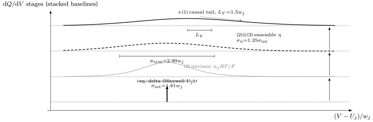
Figure 14: 두-상 broadening 의 폭 예산(식 (1.80)), 네 단계를 공유 x 축 위 계단(waterfall)으로 서사화 — 아래에서 위로 쌓아 폭이 실제로 넓어지는 것을 한눈에 비교한다(점선 = 각 단계의 기준선, 오른쪽 여백의 수직 화살표가 단계 전이). 맨 아래 굵은 화살 = 평형 델타(Maxwell 전위). 회색 = ② 내재 logistic 미분 중(폭 \sigma_{\text{int}} = 1.81w_j ). 파선 = ②⊗③ — 실제 수치 합성곱(Gaussian 예시 \sigma_\eta = 1.25\sigma_{\text{int}} )으로 얻은 결과이며 분산은 정확히 가법이다 — \sigma_{\text{sym}} = \sqrt{\sigma_{\text{int}}^2 + \sigma_\eta^2} = 2.90w_j 의 피타고라스 형태로, 본문 식 (1.80) 과 일치한다. 다만 본문이 쓰는 “같은 함수족이면 유효 scale 1.6w_j ” 지름길로 재현한 logistic 중은 이 실제 합성곱보다 peak 가 약 10% 높다(분산은 정확해도 모양까지 같은 logistic 족은 아님 — 근사의 한계를 명시해 둔다). 굵은 실선 = +① 인과 지수 꼬리( L_V = 1.5w_j , 식 (1.97) 의 인과 기억 적분으로 계산)가 중을 오른쪽으로 밀며, peak 위치가 중심에서 이동한다. 세 척도( \sigma_{\text{int}} \cdot \sigma_{\text{sym}} \cdot 꼬리 길이 L_V )는 치수선 길이로 직접 대비된다.
