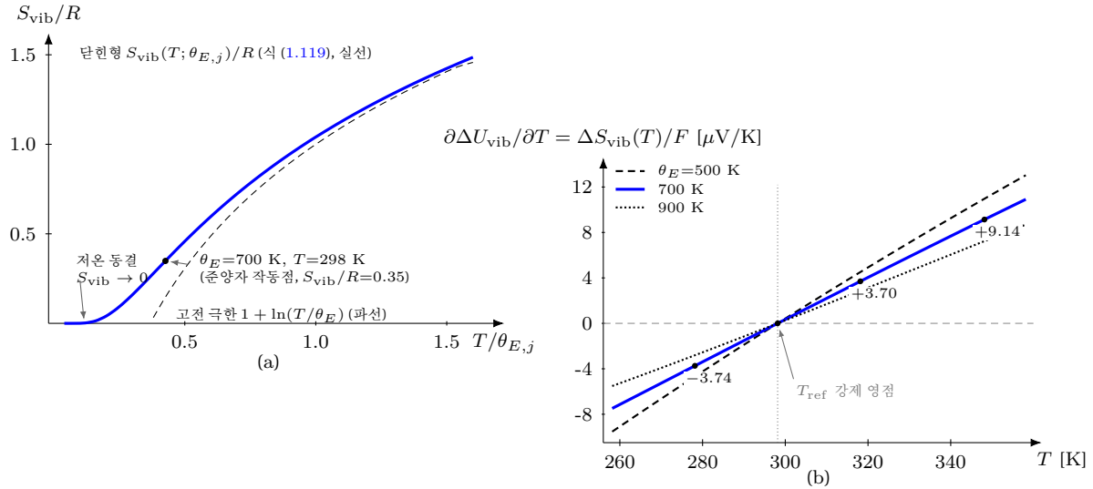
Figure 20: Einstein 진동 보정의 두 측면 — 좌표는 식 (1.119)·(1.121) 그대로의 수치 평가다. (a) 단원형 S_{\text{vib}}(T; \theta_{E,j})/R : 저온 ( u_j \rightarrow \infty ) 에서 0 으로 동결되고 고전 극한(파선) 1 + \ln(T/\theta_E) 에 T/\theta_E \gtrsim 1 에서 붙는다 — 앞 절이 중심 표준값에 흡수한 “ T -무관 상수”는 이 곡선을 T_{\text{ref}} 에서 한번 평가해 동결한 값이다. ● 는 \theta_E = 700 K·298 K 의 준양자 작동점. (b) 중심 이동의 온도 기울기 \partial \Delta U_{\text{vib}} / \partial T = \Delta S_{\text{vib}}(T) / F : \theta_E = 500/700/900 K 모두 T_{\text{ref}} 의 강제 영점을 지나 로그형 곡률로 자라며, ● 는 본문 §1.14.3 의 수치 ( \theta_E = 700 K 에서 -3.74/0/+3.70/+9.14 \mu\text{V/K} ) 다. electronic 항( \propto T )은 곡률이 0 이라 두 함수형이 다운도 곡률 피팅에서 갈리고, 분리에는 준양자 영역에 놓인 온도점 셋 이상이 필요하다.
