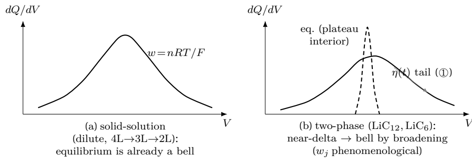
Figure 15: 평형 모양과 broadening. (a) 연속 고용체 전이 — 평형 단일 입자 dQ/dV 가 이미 폭 n_j RT/F 의 종(식 (1.76)), broadening 불요. (b) 두-상 전이 — 평형은 plateau 내부에서 거의 날카로운 선(파선; 양끝 단상 꼬리 탓에 폭이 정확히 0 은 아님)이고, 실측은 세 출처가 펼친 치우친 종(실선)이다: ① 유한율속 비대칭 꼬리 (§1.8–§1.9 의 L_V , |I| \rightarrow 0 소멸), ② 전류 무관한 가장자리 내재 폭( \sim RT/F ), ③ 길보기 중심 U_{app} = U_j + \eta 의 입자간 \eta 산포를 forward 평균한 앙상블 몫(식 (1.79)). ①의 \eta(t) (한 입자의 시간 변화)와 ③의 입자간 \eta 산포는 같은 과전압의 다른 평균이며, 평형 중심 U_j 는 입자 무관 상수다 — 분포하는 것은 \eta . 세 출처의 지위와 한정(폭 w_j 의 현상학적 지위·흑연 두-상 국한· \rho(U_{app}) 역산 금지·사이즈 배제)은 본문 §1.7.2·§1.7.3.
