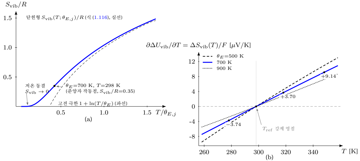
Figure 20: Einstein 진동 보정의 두 측면 — 좌표는 식 (1.116)·(1.118) 그대로의 수치 평가다. (a) 단원형 S_{\text{vib}}(T; \theta_{E,j})/R : 저온 ( u_j \rightarrow \infty ) 에서 0 으로 동결되고 고전 극한(파선) 1 + \ln(T/\theta_E) 에 T/\theta_E \gtrsim 1 에서 붙는다 — 앞 절이 중심 표준값에 흡수한 “ T -무관 상수”는 이 곡선을 T_{\text{ref}} 에서 한번 평가해 동결한 값이다. ● 는 \theta_E = 700 \text{ K} , T = 298 \text{ K} 의 준양자 작동점. (b) 중심 이동의 온도 기울기 \partial \Delta U_{\text{vib}} / \partial T = \Delta S_{\text{vib}}(T) / F : \theta_E = 500/700/900 \text{ K} 모두 T_{\text{ref}} 의 강제 영점을 지나 로그형 곡률로 자라며, ● 는 본문 §1.14.3 의 수치 ( \theta_E = 700 \text{ K} 에서 -3.74/0/+3.70/+9.14 \mu\text{V/K} ) 다. electronic 항( \propto T )은 곡률이 0 이라 두 함수형이 다운도 곡률 피팅에서 갈리고, 분리에는 준양자 영역에 놓인 온도점 셋 이상이 필요하다.
