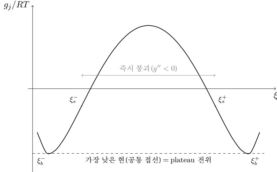
Figure 3: 가운데가 언덕이 된 자유에너지( \Omega_j = 3RT ). 곡선이 현(파선)보다 위에 있는 두 점점 \xi_b^\pm 사이에서는 갈라지는 쪽이 이득이다 — 이 경계가 binodal 이고, 접선의 기울기가 plateau 전위다. 그 안의 변곡점 \xi_s^\pm 사이( g'' < 0 )는 미소 요동에도 즉시 무너지는 불안정 영역 — 이 경계가 spinodal 이다. 둘 사이의 띠가 준안정 — 갈라지면 이득이지만 핵생성 장벽을 넘어야 하는 영역 — 이며, 충방전 히스테리시스의 무대가 된다.
