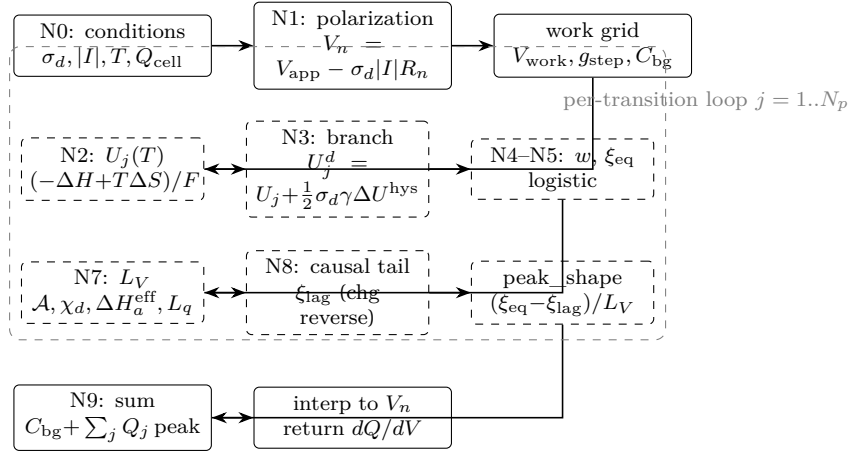
Figure 5: 한 곡선을 그리는 계산 진행 N0 \rightarrow N9 (코드 curve → dqdv ). 위 줄 = 조건 환산·분극·작업 격자( N0 – N1 ). 점선 상자 = 전이별 루프( N2 – N8 ): 평형 중심→분기→폭·점유→자연 길이→인과 꼬리→peak 모양. 아래 줄 = 합산과 측정축 역보간( N9 ). 본 장의 절 순서가 이 흐름과 1:1.
