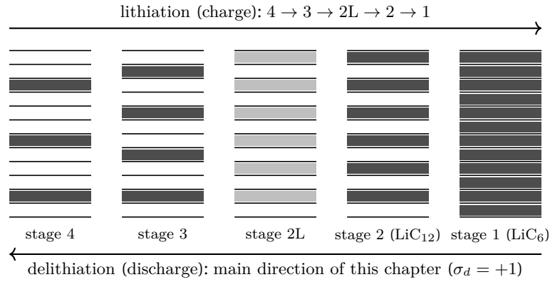
Figure 1: 흑연 staging의 갤러리 채움 도식. 수평선이 그래핀 층, 음영 띠가 리튬이 든 층간 갤러리다. 채울수록 stage 번호가 줄어 stage 1( \text{LiC}_6 , 완전 채움)에 닿고, 각 stage 전이가 dQ/dV 에 peak 하나를 남긴다. stage 2L은 갤러리 안이 희박하고 면내 질서가 풀린(liquid-like) 단계라 열게 표시했다. 코드의 전이 목록이 표 2의 네 전이( 4 \rightarrow 3 , 3 \rightarrow 2L , 2L \rightarrow 2 , 2 \rightarrow 1 )다.
