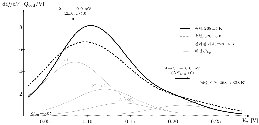
Figure 18: 합산식 (1.97) 이 내는 전체 곡선 — 좌표는 식 그대로의 수치 평가다: 초기 상태의 평형 중 전용 극한( L_V \rightarrow 0 \cdot \gamma_j = 0 \cdot R_n = 0 )에서 dQ/dV = C_{bg} + \sum_j Q_j \xi_{eq,j} (1 - \xi_{eq,j}) / w_j 를 표 2 초기값으로 평가했다( U_j(T) = (-\Delta H_{rxn,j} + T \Delta S_{rxn,j}) / F 를 온도마다 재평가, w_j = RT/F - n_j = 1 균일, 배경은 상수 예시 C_{bg} = 0.05 Q_{cell}/V ). 회색 가는 곡선이 298.15 K 의 전이별 기여, 굵은 실선·파선이 268.15/328.15 K 의 총합이다. 온도가 오르면 (i) 폭 w = RT/F 가 비례해 열려 봉우리가 낮고 넓어지고 (면적 Q_j 보존), (ii) 중심은 \partial U_j / \partial T = \Delta S_{rxn,j} / F 를 따라 전이마다 반대 방향으로 움직인다 — 60 K 동안 2 \rightarrow 1 ( \Delta S_{rxn} = -16 \text{ J}/(\text{mol K}) ) 은 -9.9 \text{ mV} 로 왼쪽, 4 \rightarrow 3 (+29) 은 +18.0 \text{ mV} 로 오른쪽(화살표), 3 \rightarrow 2L(0) 은 제자리다. 다운도 피팅에서 온도마다 U_j(T) 를 따로 읽어야 하는 까닭 (§1.3) 이 이 한장이다.
