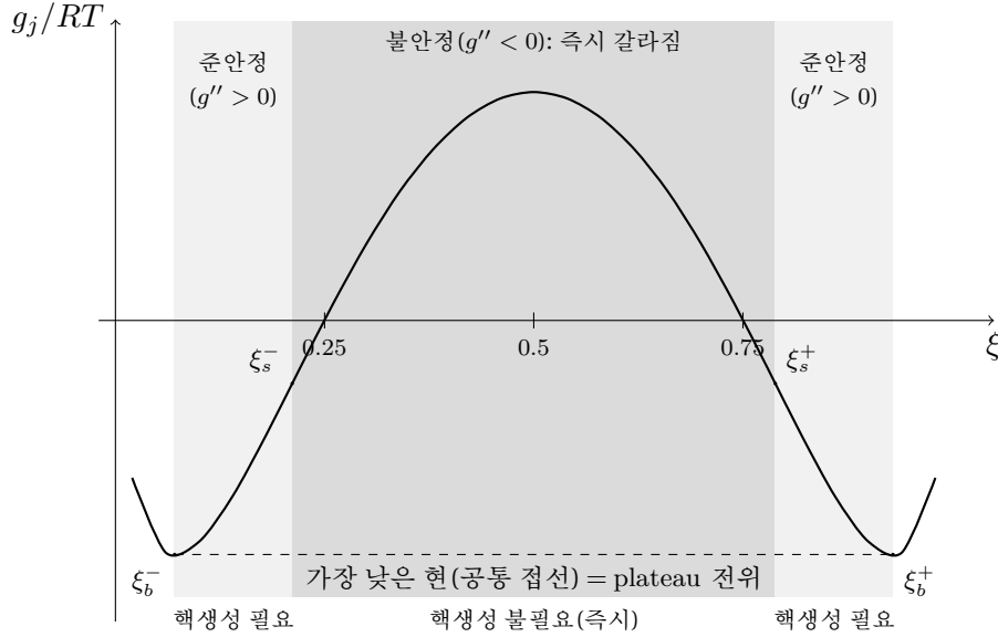
Figure 6: 가운데가 언덕이 된 자유에너지( \Omega_j = 3RT — 곡선은 식 (1.33), 띠 경계는 식 (1.40) 의 실제산값). 곡선이 현(파선)보다 위에 있는 두 점점 \xi_b^\pm 사이에서는 갈라지는 쪽이 이득이다 — 이 경계가 binodal 이고, 접선의 기울기가 plateau 전위를 정한다( g' = sF(V_{eq} - U_j) — 식 (1.38)). 진한 띠( \xi_s^- < \xi < \xi_s^+ , g'' < 0 )는 미소 요동에도 즉시 무너지는 불안정 영역 — 경계가 spinodal 이다. 얇은 띠(binodal-spinodal 사이)가 준안정 — 갈라지면 이득이지만 핵생성 장벽을 넘어야 도달하는 영역 — 이며, 충방전 히스테리시스의 무대가 된다. 띠 밖(binodal 바깥)은 균질 단상이 최선인 안정 영역이다.
