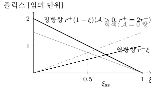
Figure 4: 정지점의 시각화(실계산). 정방향 플럭스 r^+(1-\xi) 는 차 있는 자리가 줄며 감소하는 직선, 역방향 r^-\xi 는 빈 자리가 늘며 증가하는 직선 — 교점이 정지점 (1.25) 이다. \mathcal{A} > 0 ( r^+ = 2r^- 예시, 검정 짙)이면 교점이 \xi_{ss} = 2/3 로 밀리고, \mathcal{A} = 0 (회색 짙)이면 \frac{1}{2} — 구동력이 정지점을 미치는 방식 (1.26) 그 자체다.
