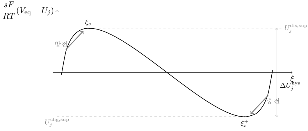
Figure 8: 비단조 평형 전위 (1.66) ( \Omega_j = 4RT ). 방전은 상승 준안정 가지를 타고 극대 \xi_s^- 까지, 충전은 반대쪽 극소 \xi_s^+ 까지 과주행한다. 두 극값의 차가 spinodal 상한 gap \Delta U_j^{hys} 이고 (위 첨자 sup 는 spinodal 상한 표시), 실측 분기는 축소 인자 \gamma_j 만큼 그 안쪽에 선다.
