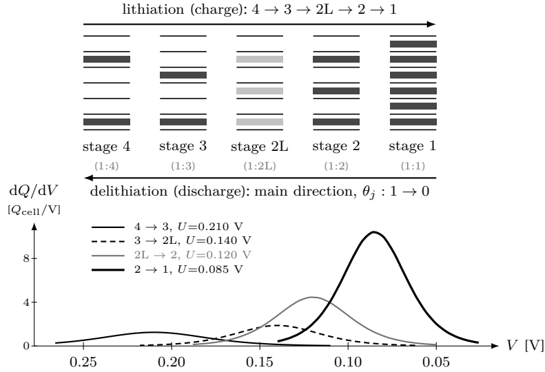
Figure 2: 흑연 staging의 갤러리 채움 도식(위)과 대응 dQ/dV peak(아래, 식 (1.61)의 초기값 수치 평가 — dQ/dV = Q_j \xi_{\text{eq}}(1 - \xi_{\text{eq}})/w_j , 표 2의 U_j, Q_j, w_j ). 위: 수평선이 그려진 층, 음영 띠가 리튬이 든 층간 갤러리다. 채울수록 stage 번호가 줄어 stage 1(LiC 6 , 완전 채움)에 닿고, 열 아래 비율(1:4→1:1)이 각 stage의 갤러리 점유 주기다. stage 2L은 면내 질서가 풀린 단계라 열게 표시했다. 아래: 네 초기값 전이의 실제 peak — 높이 Q_j/(4w_j) 는 전이마다 크게 다르다 ( 2 \rightarrow 1 이 가장 큼, 10.4 Q_{\text{cell}}/V ). 주의 — 위 갤러리 열 간격은 범주형(등간격 스케치)이고 아래 V 축은 실제 전위 스케일(비등간격 — 3 \rightarrow 2L 과 2L \rightarrow 2 은 겨우 20 mV 차이로 갤러리 열 간격에 선형 정렬되지 않는다)이라, 둘은 전이명(예 2 \rightarrow 1 )으로만 대응시킨다. 본 문건 방향은 방전(탈리튬화)이다.
