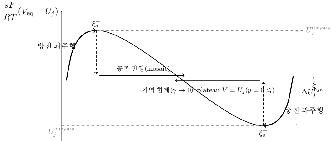
Figure 8: 비단조 평형 전위 (1.66) ( \Omega_j = 4RT )와 과주행 경로. 방전(굵은 경로, 좌상)은 상승 준안정 가지를 타고 극대 \xi_s^- 까지 과주행한 뒤, 분리가 점화되며 공존 plateau ( V = U_j , y = 0 축)로 낙하해 (점선 화살표) mosaic 공존으로 진행한다. 충전(우하)은 거울상으로 극소 \xi_s^+ 까지 과주행한다. 두 극값의 차가 spinodal 상한 gap \Delta U_j^{\text{hys}} 이고(위첨자 sup 는 spinodal 상한 표시), 실측 분기는 축소 인자 \gamma_j 만큼 그 안쪽에 선다 — \gamma \rightarrow 0 의 가역 한계에서 두 경로가 모두 y = 0 의 plateau 로 합쳐진다.
