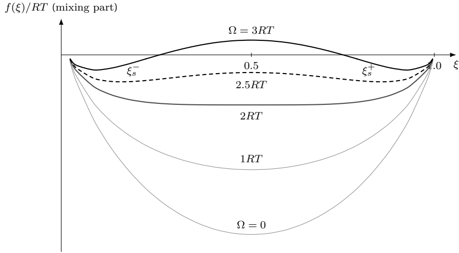
Figure 4: 정규용액 조성 자유에너지의 섞임 몫 f(\xi)/RT = \xi \ln \xi + (1-\xi) \ln(1-\xi) + (\Omega/RT) \xi(1-\xi) (좌표는 식 그대로의 수치 평가). \Omega \leq 2RT 면 한 웬, \Omega = 2RT 에서 바닥이 평탄해지고 (문턱, 식 (1.31)), \Omega > 2RT 면 가운데가 언덕이 된 이중웰 — \Omega = 3RT 곡선의 점이 spinodal \xi_s^\pm = 0.2113/0.7887 이다. 닫힌 근은 §1.4 가 닫으며, 그 절의 이중웰 그림이 이 가족 중 \Omega = 3RT 한 장을 확대한 것이다.
