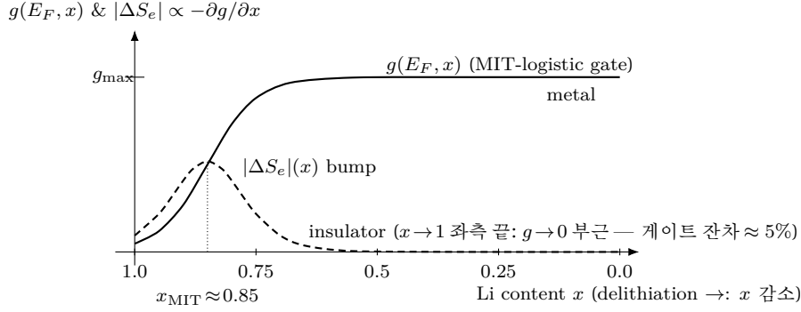
Figure 20: LCO 전자 엔트로피의 MIT-logistic 게이트. 실선 = g(E_F, x) (식 (1.123)): x \approx 1 절연체에서 \approx 0 , 탈리튬화로 x_{MIT} \approx 0.85 부근에서 metal 의 g_{max} = 13 \text{ eV/atom} 으로 커진다. 파선 = 탈리튬화 시 방출되는 부분몰 전자 엔트로피 |\Delta S_e| = -\partial S_e / \partial x \propto -\partial g / \partial x > 0 (식 (1.119)·단형식 (1.124); 삽입 기준 \Delta S_e = \partial S_e / \partial x < 0 의 절댓값으로, x_{MIT} 에서 \sigma(1 - \sigma) 가 최대): 전이 중심의 국소 봉우리다 — 작지만(게이트 골 몰당 \approx -46 \text{ J/(mol K)} , §1.15.5) MIT 구간에만 커지는 게이트라 config 단독으로 대체 불가. \Delta S_{e,j} \propto T 라 다른 항과 달리 전자 기여의 \partial U / \partial T 가 T 에 선형 (§1.15.2; U-이동은 \propto T^2 ). 흑연엔 이 봉우리가 없다( g(E_F) 변화 미미).
