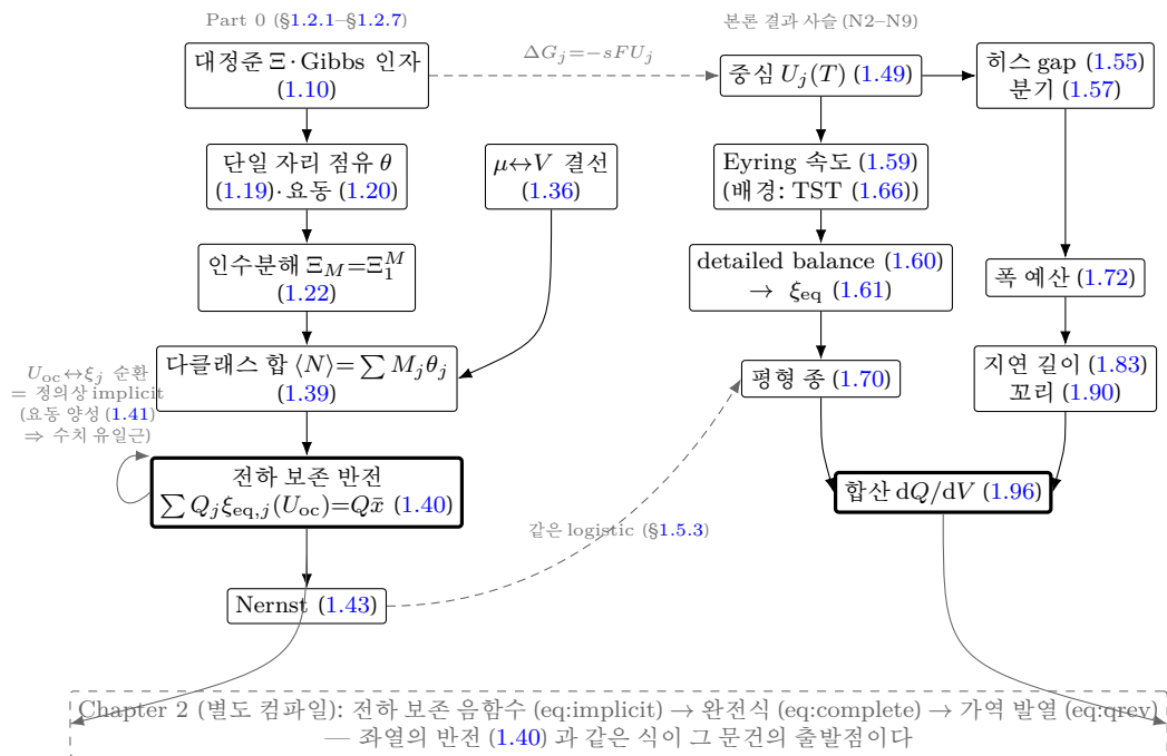
Figure 21: 식 의존성 지도(항법판 전용 도식) — 화살표는 “이 식이 저 식의 입력이다”를 뜻한다. 좌열이 Part 0 사다리, 중·우열이 본론 결과 사슬(N2–N9) 이고, 굵은 상자들(전하 보존 방전 (1.40)·합산 (1.96))이 내부 전위 결정과 관측 곡선 산출의 두 중심이다. 좌열 옆 고리는 U_{oc} 와 \xi_j 의 순환 의존이 논리 공백이 아니라 정의상 implicit formulation 이고(요동 양성 (1.41) 이 유일근을 보증), 하단 파선 상자는 별도 컴파일인 Chapter 2 로의 연계(서술형 참조)다.
