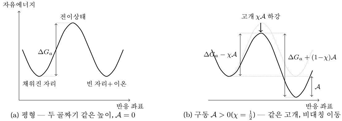
Figure 1: 활성화 장벽 그림(실계산: f_0(x) 이중 골짜기에 구동 기울임 -As(x) 를 더한 것, A = 0.39 \Delta G_a ). (a) 평형 — 두 골짜기가 같은 높이이고 사건 속도는 고개 높이 \Delta G_a 의 Boltzmann 인자에 시도 빈도 k_0 를 곱한 식 (1.1) 을 따른다. (b) 구동력 A_j 가 도착 골짜기를 A 만큼 내리면 같은 고개를 공유하는 두 방향의 장벽이 비대칭으로 변한다 — 정방향은 \Delta G_a - \chi A 로 낮아지고 역방향은 \Delta G_a + (1 - \chi)A 로 높아진다 (§1.4 식 (1.15) 의 시각 짝; 점선은 (a)의 평형 풍경). 온도는 풍경을 기울이지 않는 대신 지수의 분모( RT )로 들어와 넘는 확률 자체를 키운다(고개 높이의 엔트로피 몫 -T\Delta S_a 는 §1.10 의 절편으로 처리된다).
