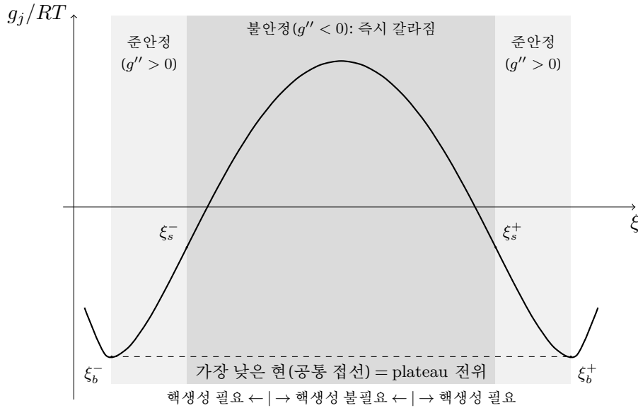
Figure 3: 가운데가 언덕이 된 자유에너지( \Omega_j = 3RT , 띠 경계는 실제산값). 곡선이 현(파선)보다 위에 있는 두 점점 \xi_b^\pm 사이에서는 갈라지는 쪽이 이득이다 — 이 경계가 binodal 이고, 접선의 기울기가 plateau 전위다. 진한 띠( \xi_s^- < \xi < \xi_s^+ , g'' < 0 )는 미소 요동에도 즉시 무너지는 불안정 영역 — 경계가 spinodal 이다. 옅은 띠 띠(binodal-spinodal 사이)가 준안정 — 갈라지면 이득이지만 핵생성 장벽을 넘어야 도달하는 영역 — 이며, 충방전 히스테리시스의 무대가 된다. 띠 밖(binodal 바깥)은 균질 단상이 최선인 안정 영역이다.
