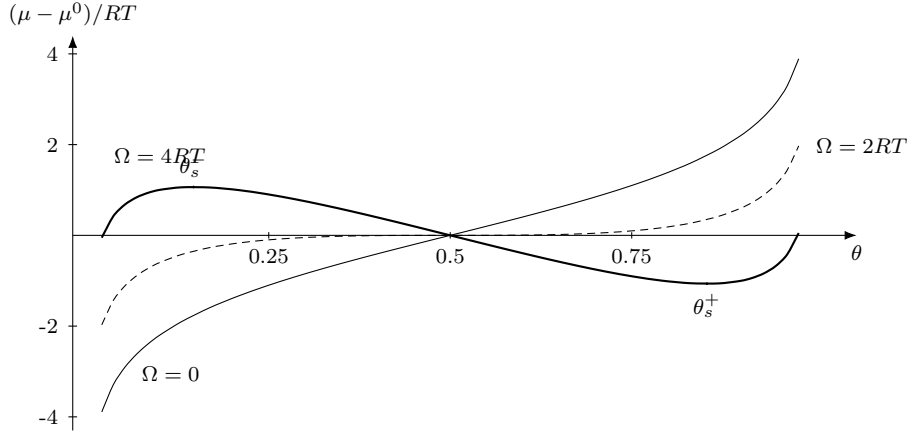
Figure 5: 격자기체 화학퍼텐셜 (\mu(\theta) - \mu^0)/RT = \ln[\theta/(1-\theta)] + (\Omega/RT)(1-2\theta) 의 개형(식 (1.19); 신규 그림 — 좌표는 식 그대로의 수치 평가). \Omega = 0 단조(로그 뭉이 양끝을 잠금), \Omega = 2RT 에서 중심 기울기 0(문턱, 식 (1.21)), \Omega = 4RT 는 비단조 — 한 \mu 에 세 \theta 가 대응하는 van der Waals loop이고 극값(점)이 spinodal \theta_s^\pm = 0.146/0.854 , 값 \pm 1.066 . §1.5 과주행 그림의 V_{eq}(\xi) 곡선은 이 곡선의 \theta = 1 - \xi 부호 반전 거울이라 같은 \pm 1.066 이 나타난다.
