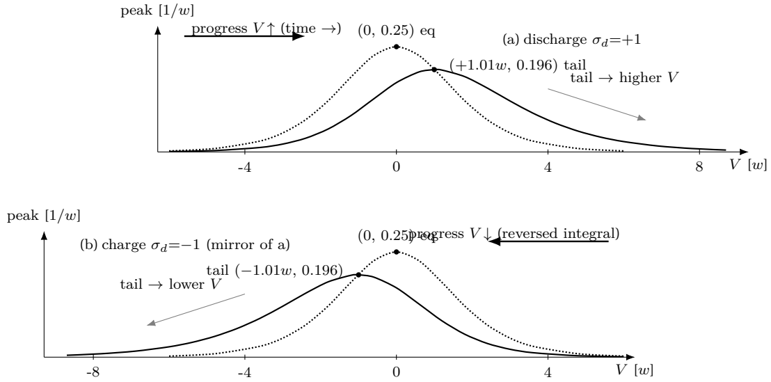
Figure 15: 인과 꼬리의 방향 — 좌표는 식 (1.89)·(1.95)의 점별 적분을 수치 평가한 값이다( w=1 , L_V=1.5w ). 점선 = 평형 중 \xi_{eq}(1 - \xi_{eq})/w (정점 0.25@중심, 방향 불변), 실선 = peak shape ( \xi_{eq} - \xi_{lag} )/ L_V (식 (1.90)). (a) 방전은 진행이 V \uparrow 라 꼬리가 높은 V 쪽으로, 정점 (+1.01w, 0.196) (식 (1.95) 상단 분기). (b) 충전은 진행이 V \downarrow 라 인과 적분이 향하는 쪽이 뒤집혀(식 (1.95) 하단 분기) 꼬리가 낮은 V 쪽으로, 정점 (-1.01w, 0.196) — 방전의 정확한 거울. 두 경우 모두 peak 는 양수. (좌표는 기억 적분의 도식 수치평가다.)
