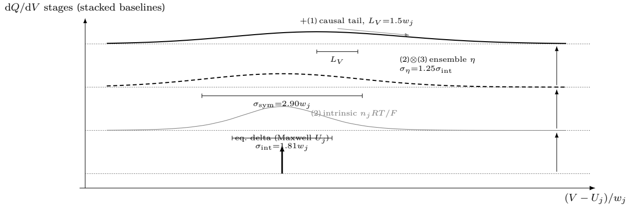
Figure 12: 두-상 broadening 의 폭 예산(식 (1.72)), 네 단계를 공유 x 축 위 계단(waterfall)으로 서사화 — 아래에서 위로 쌓아 폭이 실제로 넓어지는 것을 한눈에 비교한다(점선 = 각 단계의 기준선, 오른쪽 여백의 수직 화살표가 단계 전이). 맨 아래 굵은 화살 = 평형 델타(Maxwell 전위). 회색 = ② 내재 logistic 미분 중(폭 \sigma_{\text{int}} = 1.81w_j ). 파선 = ②⊗③ — 실제 수치 합성곱(Gaussian 예시 \sigma_{\eta} = 1.25\sigma_{\text{int}} ) 으로 얻은 결과이며 분산은 정확히 가법이다 — \sigma_{\text{sym}} = \sqrt{\sigma_{\text{int}}^2 + \sigma_{\eta}^2} = 2.90w_j 의 피타고라스 형태로, 본문 식 (1.72) 과 일치한다. 다만 본문이 쓰는 “같은 함수족이면 유효 scale 1.6w_j ” 지름길로 재현한 logistic 중은 이 실제 합성곱보다 peak 가 약 10% 높다(분산은 정확해도 모양까지 같은 logistic 족은 아님 — 근사의 한계를 명시해 둔다). 굵은 실선 = +① 인과 지수 꼬리( L_V = 1.5w_j , 식 (1.89) 의 인과 기억 적분으로 계산)가 종을 오른쪽으로 밀며, peak 위치가 중심에서 이동한다. 세 척도( \sigma_{\text{int}} \cdot \sigma_{\text{sym}} \cdot 꼬리 길이 L_V )는 치수선 길이로 직접 대비된다.
