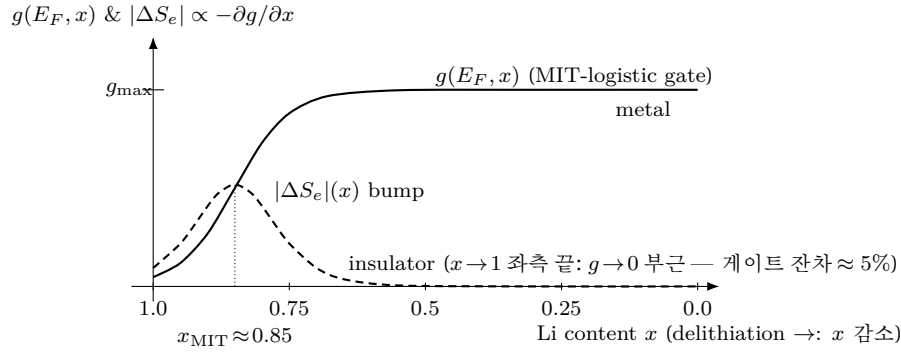
Figure 17: LCO 전자 엔트로피의 MIT-logistic 게이트. 실선 = g(E_F, x) (식 (1.123)): x \approx 1 절연체에서 \approx 0 , 탈리튬화로 x_{MIT} \approx 0.85 부근에서 metal 의 g_{max} = 13 \text{ eV/atom} 으로 커진다. 파선 = 탈리튬화 시 방출되는 부분물 전자 엔트로피 |\Delta S_e| = -\partial S_e / \partial x \propto -\partial g / \partial x > 0 (식 (1.119)·단편식 (1.124); 삽입 기준 \Delta S_e = \partial S_e / \partial x < 0 의 절댓값으로, x_{MIT} 에서 \sigma(1 - \sigma) 가 최대): 전이 중심의 국소 봉우리다 — 작지만(게이트 골 몰당 \approx -46 \text{ J/(mol K)} , §1.15.5) MIT 구간에만 커지는 게이트라 config 단독으로 대체 불가. \Delta S_{e,j} \propto T 라 다른 항과 달리 전자 기여의 \partial U / \partial T 가 T 에 선형 (§1.15.2; U-이동은 \propto T^2 ). 흑연엔 이 봉우리가 없다( g(E_F) 변화 미미).
