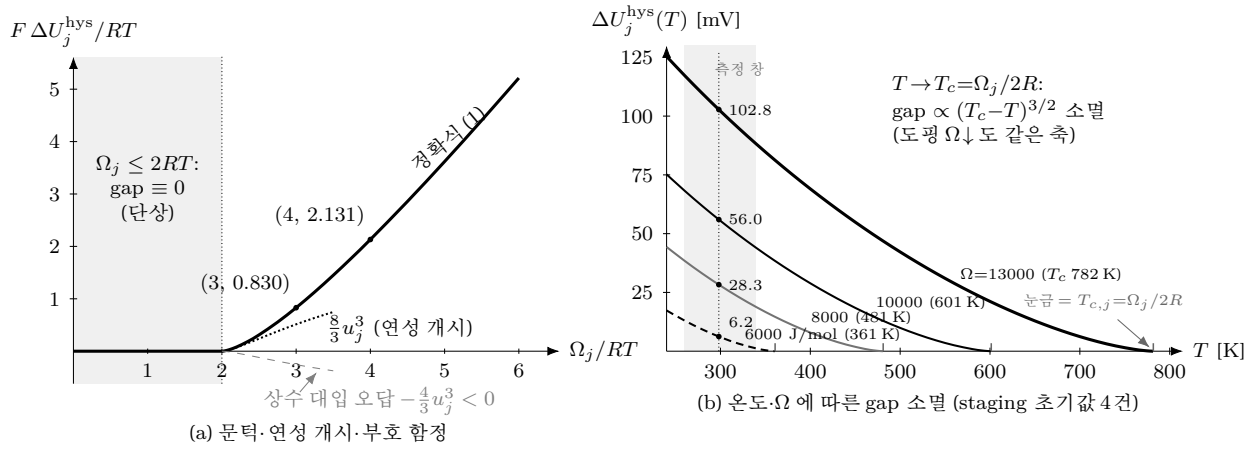
Figure 2: 히스테리시스 gap 닫힌 꼴 \Delta U_j^{\text{hys}} (식 (1))의 전 거동 — 좌표는 식 그대로의 수치 평가. (a) 무차원 gap F \Delta U_j^{\text{hys}} / RT = 2[\omega u_j - 2 \operatorname{artanh} u_j] ( \omega \equiv \Omega_j / RT , u_j = \sqrt{1 - 2/\omega} ): 문턱 \Omega_j \leq 2RT (음영)에서 정확히 0, 문턱 직후 두 급수를 함께 전개한 \frac{8}{3}u_j^3 (점선)으로 양수 연성 개시하며, \Omega_j 를 상수 대입만 한 잘못된 전개는 -\frac{4}{3}u_j^3 (회색 파선)로 부호가 뒤집힌다 (§1의 Taylor 합정). 점 (4, 2.131)은 그림 1의 \Omega_j = 4RT gap과 같은 값이다. (b) 표 1의 \Omega_j 초기값 4건을 mV로 평가한 \Delta U_j^{\text{hys}}(T) : 각 곡선은 자기 임계온도 T_{c,j} = \Omega_j / 2R (축 눈금)에서 (T_c - T)^{3/2} 로 매끄럽게 소멸한다 — 승온과 도평에 의한 \Omega_j 감소(식 (2))가 같은 축 위에서 gap을 닫는 두 손잡이다. 점선 수직선은 298.15 K, 그 교점 수치는 spinodal 상한 gap이며 실측 분기는 \gamma_j 배 안쪽이다 (식 (3)).
