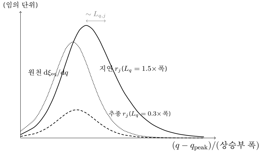
Figure 5: 일반해의 기억 거동(실계산, 두 케이스). 점선은 원천(평형 목표의 변화율). 파선은 L_q = 0.3 \times 상승부 폭 — 지연이 식 (1.44) 그대로 L_q d\xi_{eq}/dq 로 원천을 축소 추종하고(정점 높이 \approx L_q \times 원천 정점), 정점 이동도 커널 평균 \sim L_q (식 (1.63))에 머문다. 실선은 L_q = 1.5 \times 폭 — 기억이 상승부를 통째로 덮어 정점이 원천보다 낮고 높으며, 원천이 포화로 꺼진 뒤에는 식 (1.45)의 순수 지수 감쇠로 넘어간다. 상승부 극한(추종)과 꼬리 극한(지수 기억)이 같은 일반해 (1.42)의 두 얼굴임을 한 그림으로 보였다.
