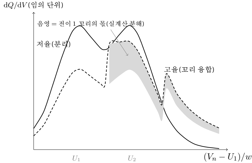
Figure 8: 두 인접 전이의 융합(중심 간격 3.9w ). 실선은 저울( r_a \rightarrow 0 ) — 골이 깊어 분리가 일어난다. 파선은 고울( r_a = 0.35 , L_V = 4w ) — 식 (1.64) 그대로, 중 항이 (1 - r_a) = 0.65 로 깎이고 각 전이의 꼬리가 다음 전이 쪽으로 뻗어 골의 우측을 메우고 뒤 어깨를 들어 올리므로 분리 판독이 지워진다. 음영 때가 그 주변 — 고울 곡선에서 전이 1 꼬리가 보태는 뭉(실계산 분해: 진폭 r_a/L_V = 0.0875 의 지수) — 이며, 골 위와 전이 2의 어깨 위에 걸쳐 있는 것이 보인다. 저온도 같은 방향으로 작용한다.
