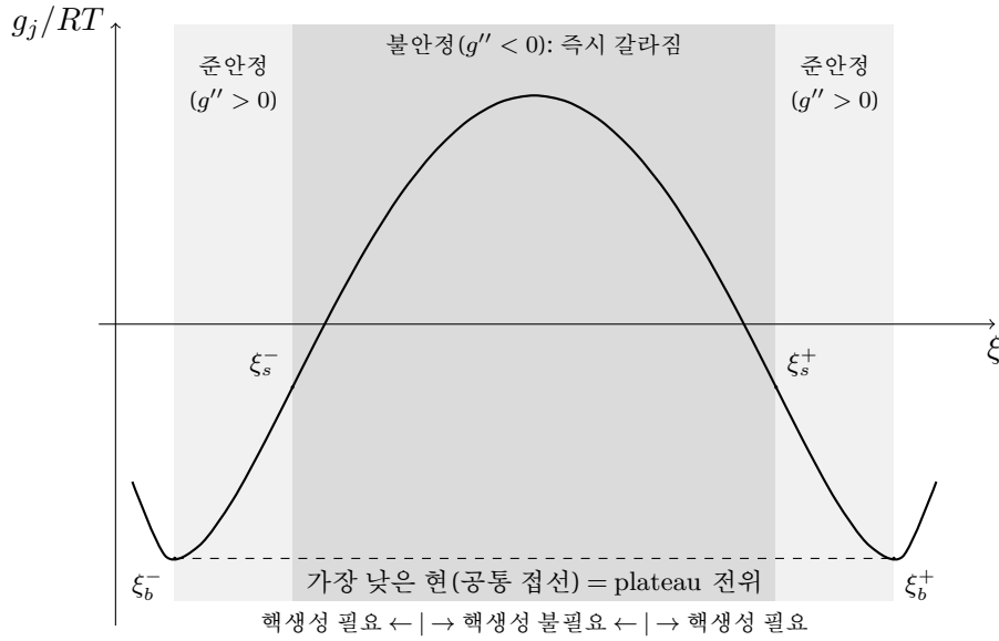
Figure 4: 가운데가 언덕이 된 자유에너지( \Omega_j = 3RT , 띠 경계는 실제산값). 곡선이 현(파선)보다 위에 있는 두 접점 \xi_b^\pm 사이에서는 갈라지는 쪽이 이득이다 — 이 경계가 binodal 이고, 접선의 기울기가 plateau 전위다. 진한 띠( \xi_s^- < \xi < \xi_s^+ , g'' < 0 )는 미소 요동에도 즉시 무너지는 불안정 영역 — 경계가 spinodal 이다. 옅은 띠 띠(binodal-spinodal 사이)가 준안정 — 갈라지면 이득이지만 핵생성 장벽을 넘어야 도달하는 영역 — 이며, 충방전 히스테리시스의 무대가 된다. 띠 밖(binodal 바깥)은 균질 단상이 최선인 안정 영역이다.
