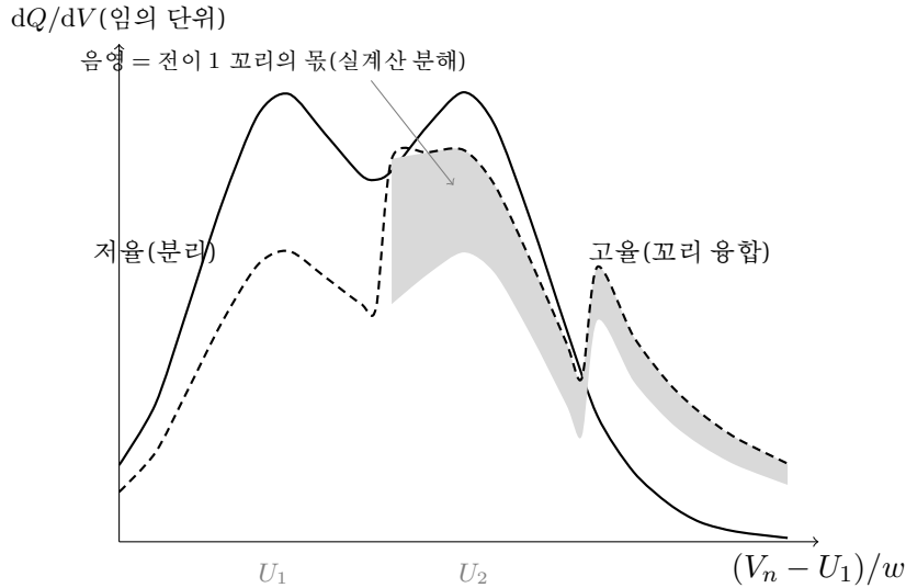
Figure 8: 두 인접 전이의 융합(중심 간격 3.9w ). 실선은 저울( r_a \rightarrow 0 ) — 골이 깊어 분리가 일어난다. 파선은 고울( r_a = 0.35 , L_V = 4w ) — 식 (1.74) 그대로, 중 항이 (1 - r_a) = 0.65 로 깎이고 각 전이의 꼬리가 다음 전이 쪽으로 뺄어 골의 우측을 매우고 뒤 어깨를 들어 올리므로 분리 판독이 지워진다. 음영 띠가 그 주변 — 고울 곡선에서 전이 1 꼬리가 보태는 뒤편(실계산 분해: 진폭 r_a/L_V = 0.0875 의 지수) —이며, 골 위와 전이 2의 어깨 위에 걸쳐 있는 것이 보인다. 저온도 같은 방향으로 작용한다.
